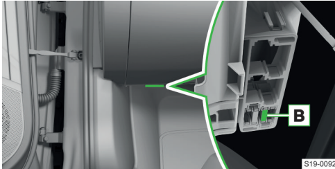
Zusatzsicherungen unter dem Ablagefach auf der Beifahrerseite für Rechtslenker
