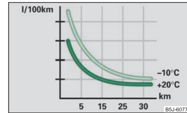
Abb. 131 Kraftstoffverbrauch in l/100 km bei verschiedenen Temperaturen
