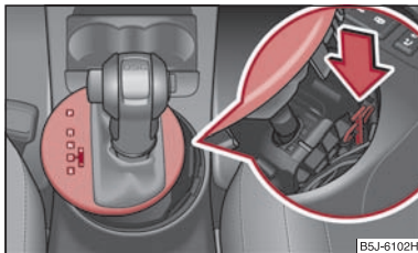
Abb. 99 Wählhebel-Notentriegelung
