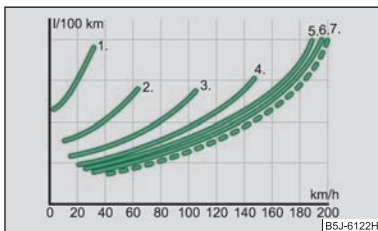
Abb. 129 Kraftstoffverbrauch in l/100 km und Geschwindigkeit in km/h
