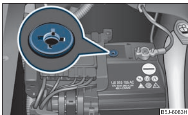
Abb. 141 Batterie: Anzeige Elektrolytstand
