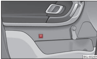
Abb. 31 Taste für Innenraumüberwachung und Abschleppschutzüberwachung
