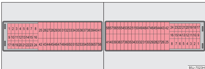
Abb. 159 Schematische Darstellung der Sicherungsbox für Links- / Rechtslenkerfahrzeuge
