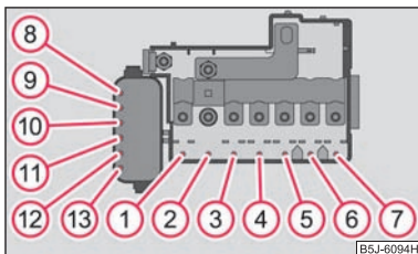
Abb. 161 Schematische Darstellung der Sicherungsbelegung an der Batterie
