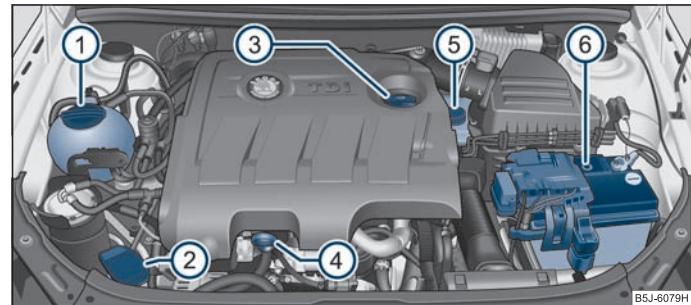
Abb. 136 Dieselmotor 1,6 l/77 kW
