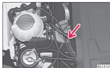
Abb. 155 Starthilfe bei Fahrzeugen mit START-STOPP-System
