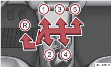
Abb. 92 Schaltschema bei Fahrzeugen mit 5-Gang Schaltgetriebe
