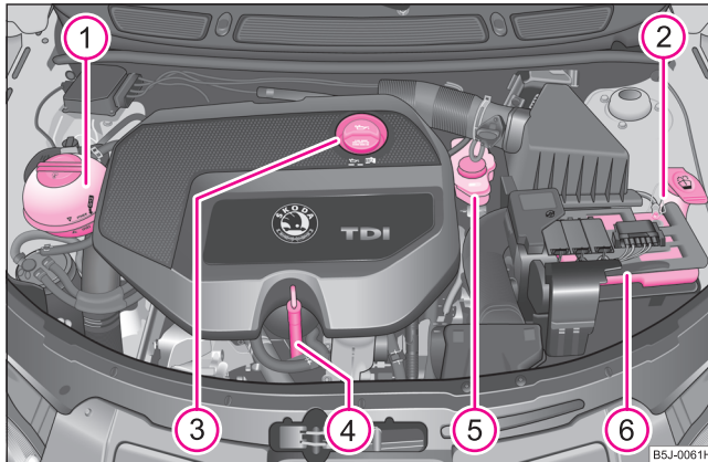
Abb. 144 Dieselmotor 1,9 l/77 kW
