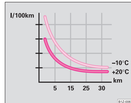
Abb. 138 Kraftstoffverbrauch in l/100 km bei verschiedenen Temperaturen
