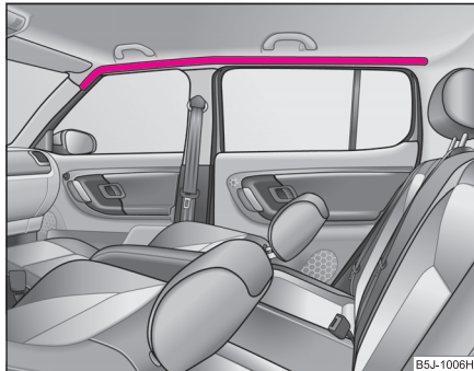
Abb. 119 Einbauort des Kopf-Airbags
