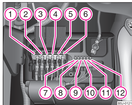
Abb. 170 Schematische Darstellung der Sicherungsbelegung an der Batterie
