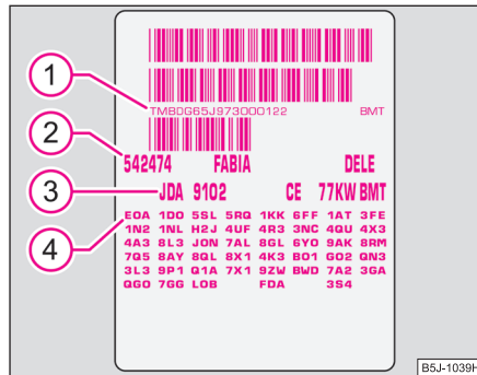
Abb. 182 Fahrzeugdatenträger
