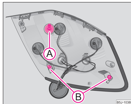
Abb. 179 Heckleuchteneinheit einbauen
