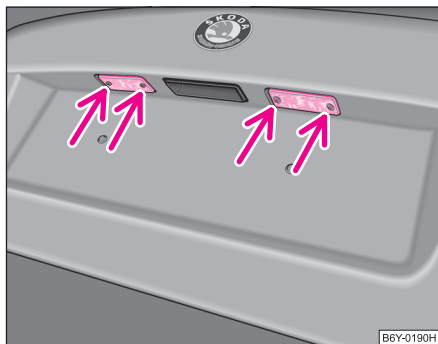
Abb. 177 Kennzeichenleuchte ausbauen
