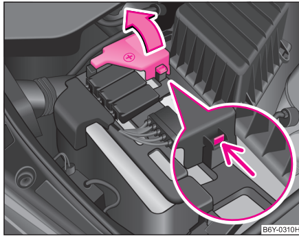
Abb. 148 Batterie: Abdeckung aufklappen
