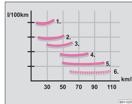
Abb. 136 Kraftstoffverbrauch in l/100 km und Geschwindigkeit in km/h
