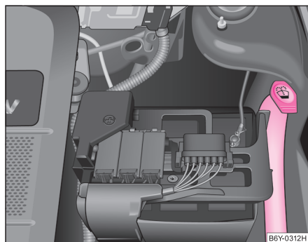
Abb. 150 Motorraum: Scheibenwaschbehälter
