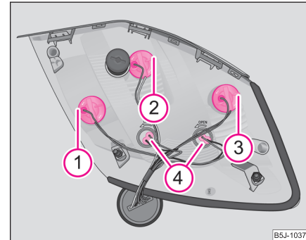
Abb. 180 Heckleuchteinheit: Einbaulage der Glühlampen
