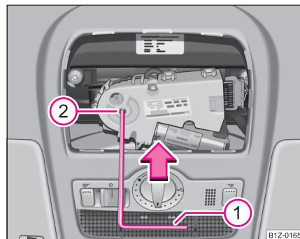
Abb. 33 Ausschnitt aus dem Dachhimmel: Notbetätigung
