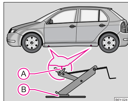
Abb. 157 Radwechsel: Ansetzstellen für den Wagenheber
