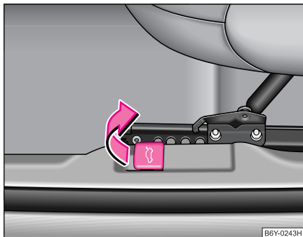
Abb. 25 Entriegelungshebel für Gepäckraumklappe
