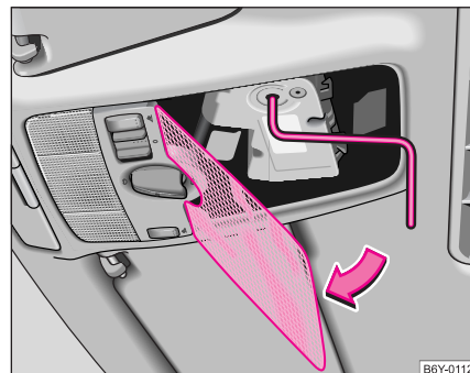
Abb. 31 Ausschnitt aus dem Dachhimmel: Notbetätigung
