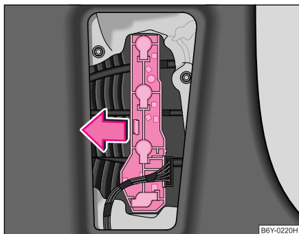
Abb. 176 Glühlampenträger ausbauen (Combi, Sedan)
