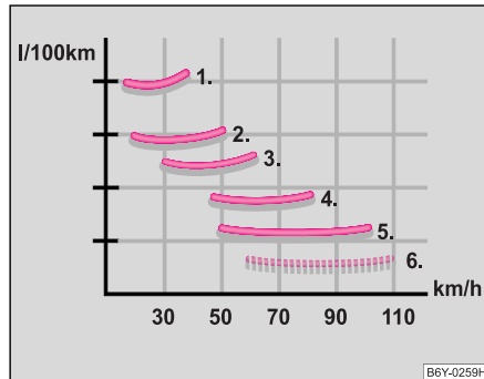
Abb. 128 Kraftstoffverbrauch in l/100 km und Geschwindigkeit in km/h
