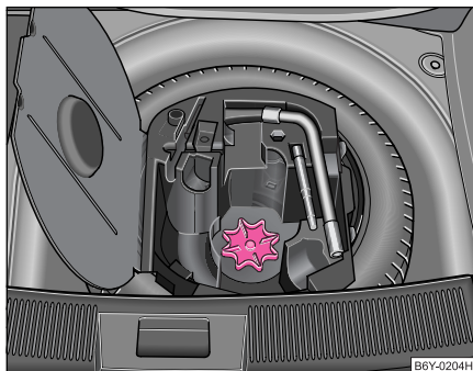
Abb. 152 Gepäckraum: Reserverad
