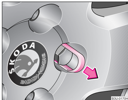
Abb. 155 Radwechsel: Abdeckkappe abnehmen
