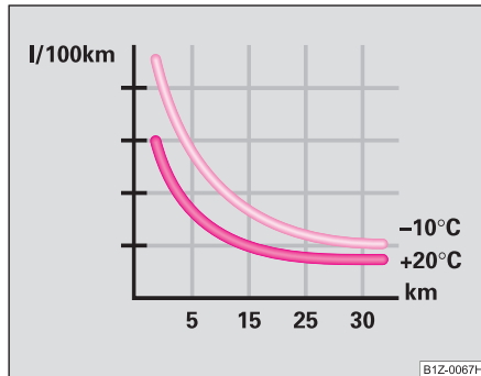
Abb. 130 Kraftstoffverbrauch in l/100 km bei verschiedenen Temperaturen
