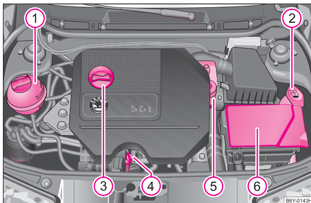
Abb. 137 Dieselmotor 1,9 l/47 kW
