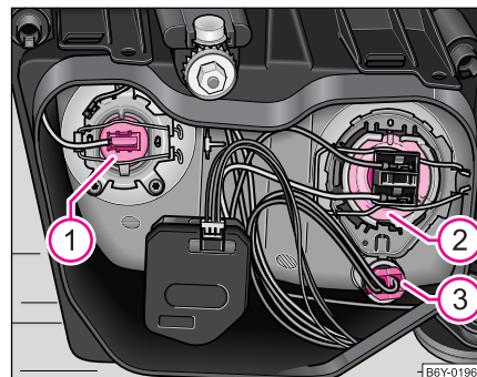
Abb. 166 Scheinwerfer vorn: Einbaulage der Glühlampen
