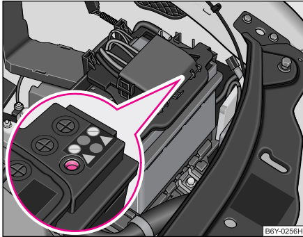
Abb. 144 Batterie mit Ladezustand-Indikator
