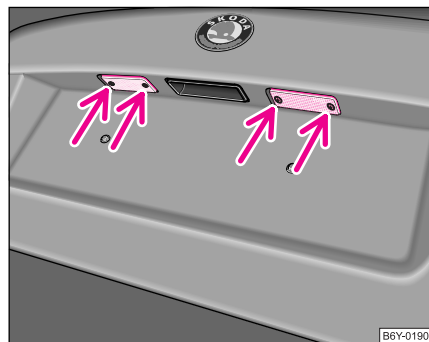
Abb. 173 Kennzeichenleuchte ausbauen
