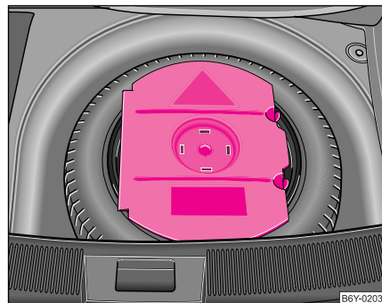
Abb. 150 Gepäckraum: Ablage für das Bordwerkzeug
