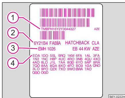
Abb. 179 Fahrzeugdatenträger
