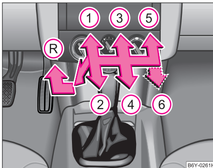
Abb. 91 Schalt-schema: 5-Gang bzw. 6-Gang Schaltgetriebe
