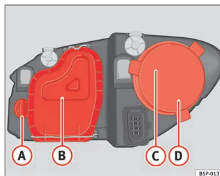
Abb. 176 Glühlampen des Hauptscheinwerfers ▶
