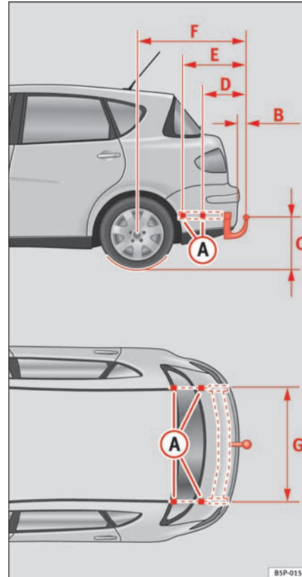
Abb. 151 Befestigungspunkte für die Anhangervorrichtung
