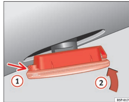
Abb. 190 Seitlicher Blinker
