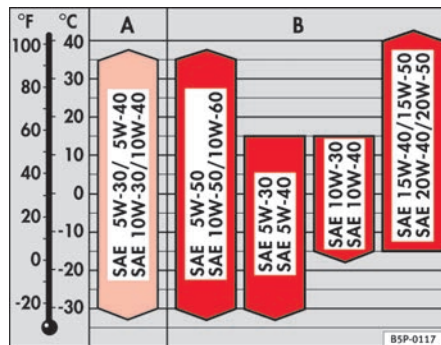
Abb. 155 Öltypen nach Temperaturbereichen
