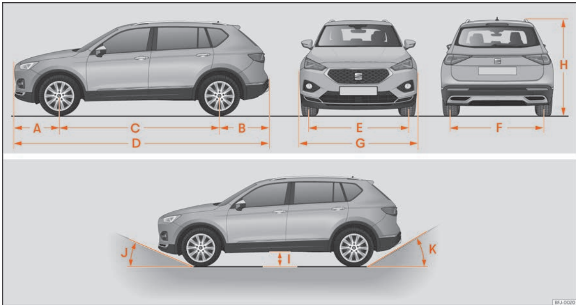
Abb. 259 Abmessungen
