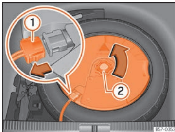
Abb. 255 Im Gepäckraum: Subwoofer ausbauen.
