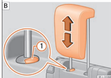
Abb. 107 Hintere Kopfstützen einstellen: A Zweite Sitzreihe, B dritte Sitzreihe.
