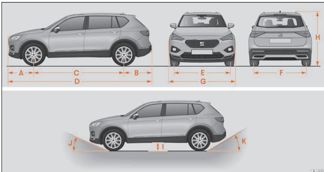
Abb. 256 Abmessungen
