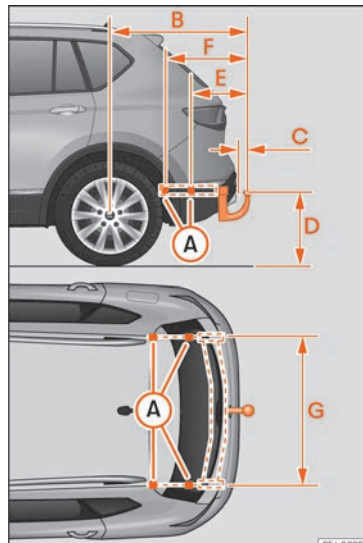
Abb. 221 Maße und Befestigungspunkte für den nachträglichen Einbau einer Anhängervorrichtung
