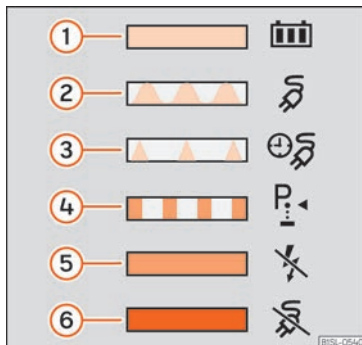
Abb. 229 Auf der Innenseite der Batterieladeklappe: Aufkleber mit Informationen zur Ladevorgangsanzeige.
