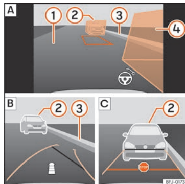
Abb. 218 Anzeige auf dem Bildschirm des Infotainment-Systems: Rückfahrassistent, Modus 2.
