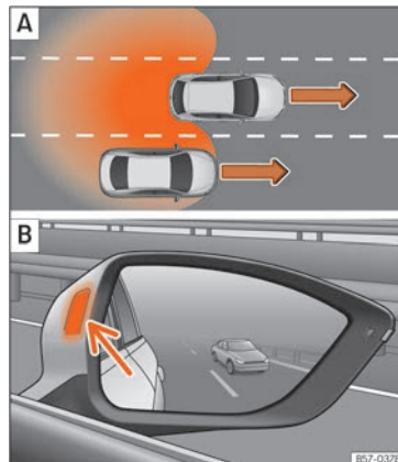
Abb. 197 Schematische Darstellung: [A] Überholvorgang und anschließender Wechsel auf die rechte Fahrbahn. [B] Anzeige des Spurwechselassistenten im Außenspiegel rechts.
