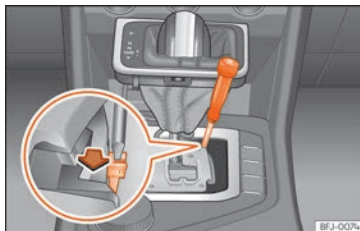
Abb. 170 Wählhebel: Notentriegeln aus der Parkstellung.
