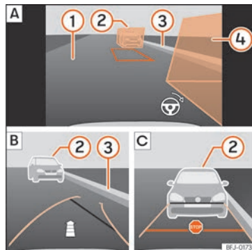
Abb. 217 Anzeige auf dem Bildschirm des Infotainment-Systems: Rückfahrassistent, Modus 2.
