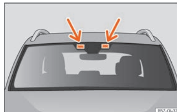
Abb. 151 Bereiche für das Anbringen elektronischen Zubehörs
