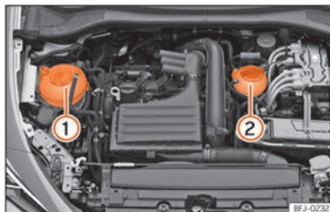
Abb. 244 Motorraum: Kühlmittelbehälter
