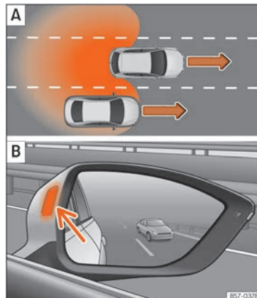
Abb. 196 Schematische Darstellung: [A] Überholvorgang und anschließender Wechsel auf die rechte Fahrbahn. [B] Anzeige des Spurwechselassistenten im Außenspiegel rechts.
