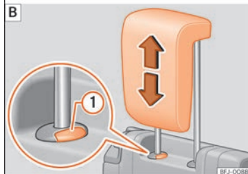
Abb. 108 Hintere Kopfstützen einstellen: A Zweite Sitzreihe, B dritte Sitzreihe.
