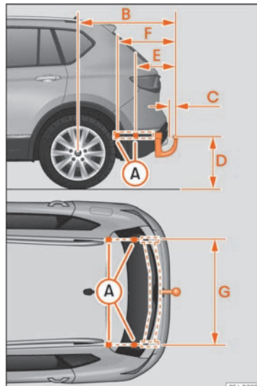
Abb. 220 Maße und Befestigungspunkte für den nachträglichen Einbau einer Anhängervorrichtung
