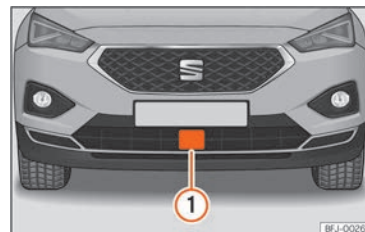
Abb. 173 Am vorderen Stoßfänger: Radarsensor.
