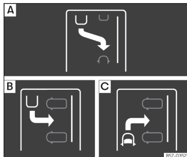
Abb. 202 Am Bildschirm des Kombi-Instruments: Anzeige der Parkmodi.
