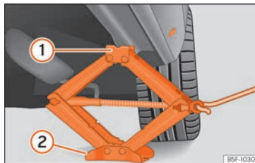
Abb. 38 Längsträger: Wagenheber ansetzen.
