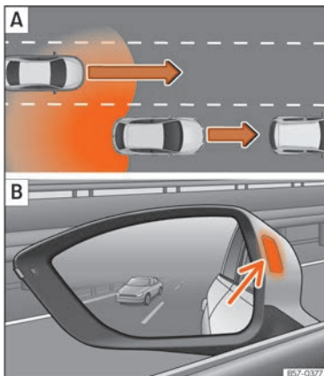
Abb. 195 Schematische Darstellung: [A] Überholvorgang mit Verkehr im hinteren Bereich. [B] Anzeige des Spurwechselassistenten im Außenspiegel links.
