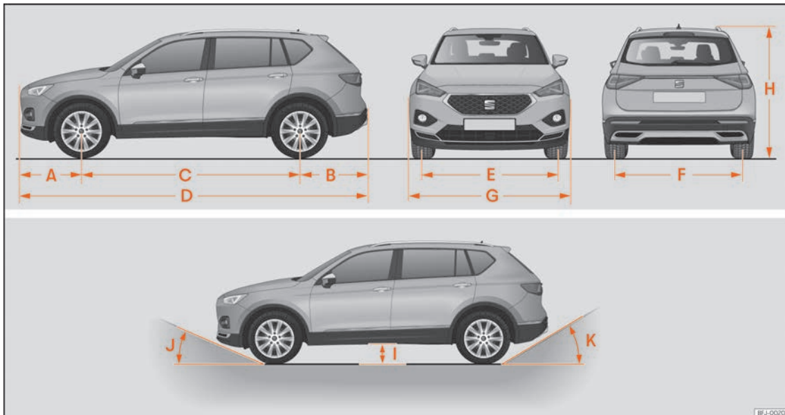
Abb. 257 Abmessungen
