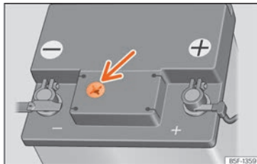
Abb. 165 Sichtfenster an der Oberseite der 12-Volt-Fahrzeuggatterie (Prinzipdarstellung).
