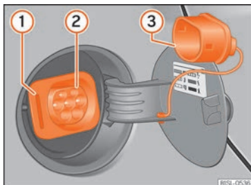
Abb. 149 Hinter der Batterieladeklappe: Ladedose (Prinzipdarstellung).
