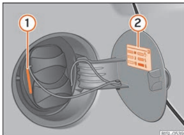
Abb. 154 Hinter der Batterieladeklappe: Ladevorgangsanzeige ① und Informationen auf dem Aufkleber ②.
