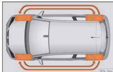
Abb. 168 Räder tauschen
