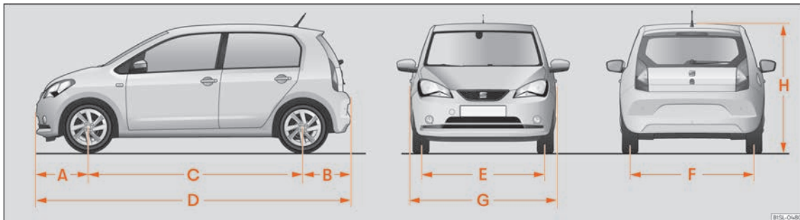
Abb. 170 Abmessungen
