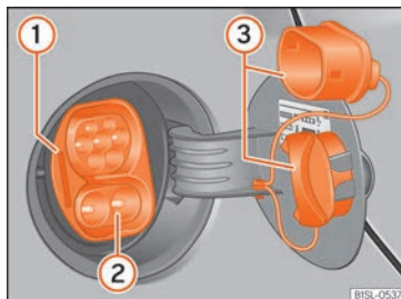
Abb. 151 Hinter der Batterieladeklappe: Ladedose (Prinzipdarstellung).
