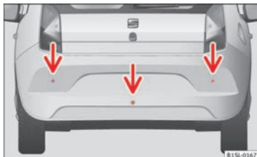
Abb. 85 Sensoren der Parkdistanzkontrolle im hinteren Stoßfänger.
