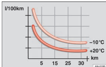
Abb. 84 Kraftstoffverbrauch in l/100 km bei 2 verschiedenen Umgebungstemperaturen.
