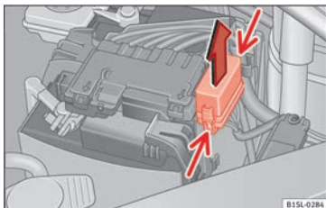
Abb. 144 Im Motorraum: Abdeckung des Sicherungskastens.
