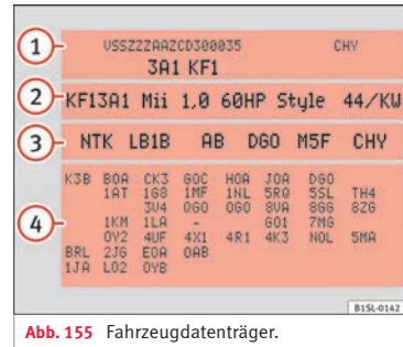
Abb. 155 Fahrzeugdatenträger.
