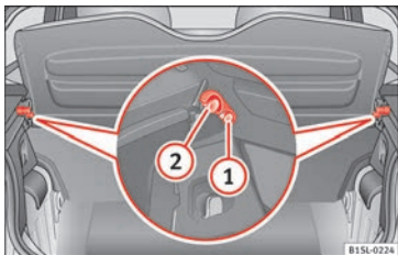
Abb. 70 Im Gepäckraum: Gepäckraumabdeckung aus- und einbauen.
