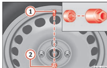
Abb. 128 Radwechsel: Reifenventil 1 und Einbautort der Anti-Diebstahl-Radschraube 2 .
