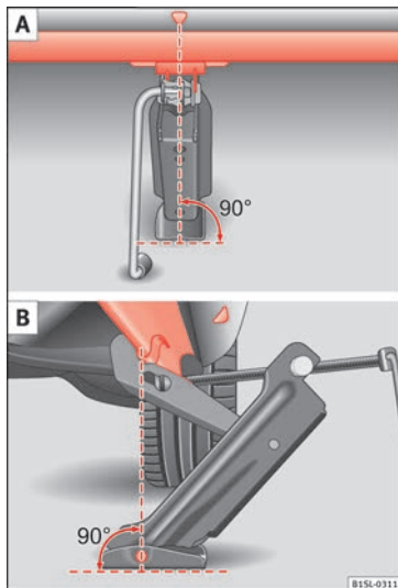
Abb. 130 Wagenheber hinten an der linken Fahrzeugseite angesetzt.
