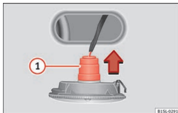
Abb. 154 Seitliche Blinkleuchte: Glühlampentausch.
