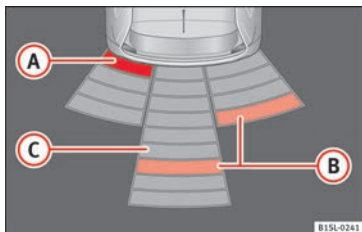
Abb. 86 Bildschirmanzeige des OPS: A Hindernis im Kollisionsbereich erkannt. B Hindernis im Segment erkannt. C Abgetasteter Bereich hinter dem Fahrzeug.
