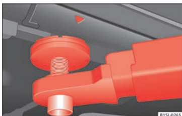
Abb. 97 Aufnahmepunkte hinten zum Anheben mit der Hebebühne oder dem Wagenheber.
