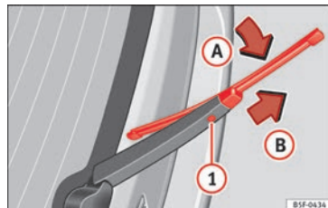
Abb. 142 Scheibenwischerblatt der Heckscheibe austauschen.
