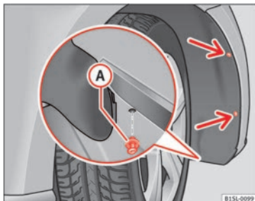
Abb. 147 Im Radhaus vorn rechts: Befestigungsschrauben (Pfeile) herausdrehen und Spreizniet A entfernen.
