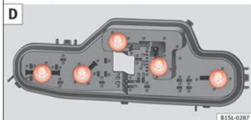
Abb. 150 Rückleuchte: C: Lampenhalter ausbauen, D: Lampen ausbauen.
