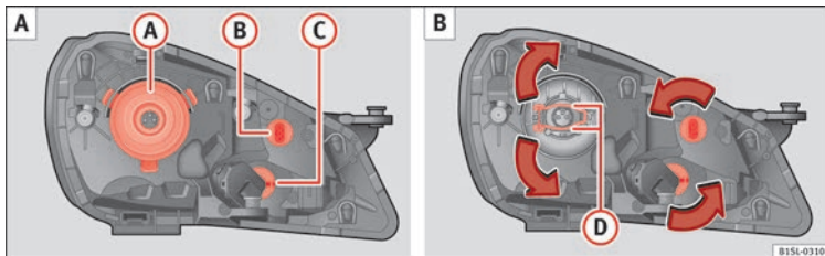
Abb. 146 Im Motorraum: Rückansicht des linken Frontscheinwerfers mit Gummiabdeckung: A Abblendlicht und Fernlicht, B Standlicht und Tagfahrlicht, C Blinklicht.
