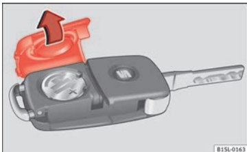
Abb. 30 Fahrzeugschlüssel: Deckel für Batteriefach.
