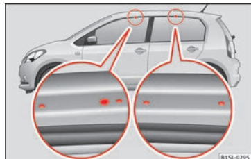
Abb. 75 Befestigungspunkte für Grundträger und Dachgepäckträger in 4-türigen Fahrzeugen.
