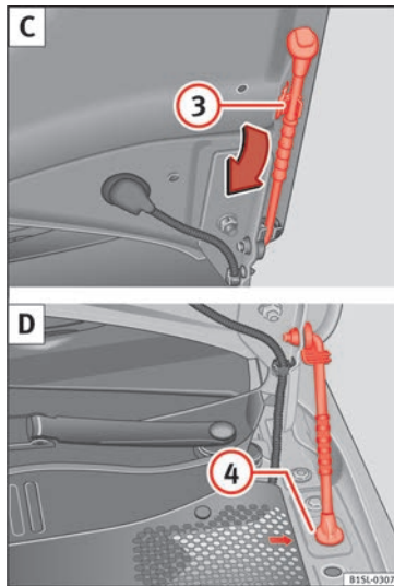
Abb. 106 C: Klappenstütze an der Motorraumklappe. D: Mit der Klappenstütze gesicherte Motorraumklappe.
