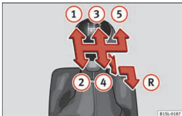
Abb. 81 Schaltschema des 5-Gang-Schaltgetriebes.
