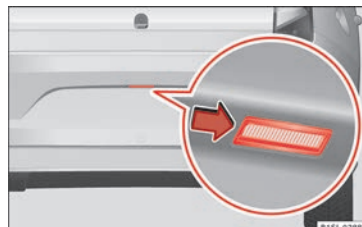
Abb. 151 Im Stoßfänger hinten: Kennzeichenleuchte ausbauen.
