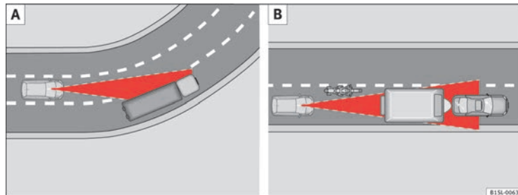
Abb. 102 A: Fahrzeug im Bereich einer Kurve. B: Vorausfahrender Motorradfahrer außerhalb des Wirkungsbereichs des Lasersensors.
