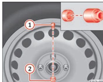
Abb. 145 Radwechsel: Reifenventil (1) und Einbaupunkt der Anti-Diebstahl-Radschraube (2).
