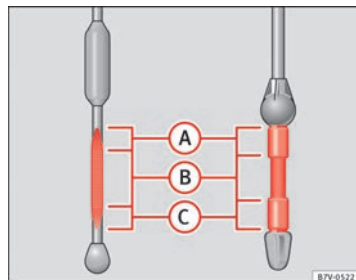
Abb. 114 Ölmeßstab mit Motorölstandsmarkierungen.
