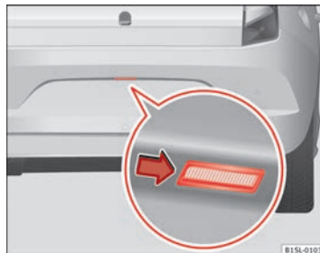
Abb. 158 Im Stoßfänger hinten: Kennzeichenleuchte ausbauen.
