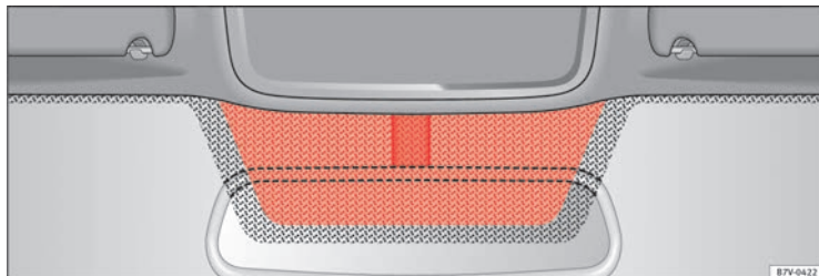
Abb. 59 Metallbeschichtete Infrarot-Frontscheibe mit Kommunikationsfenster (rote Fläche).
