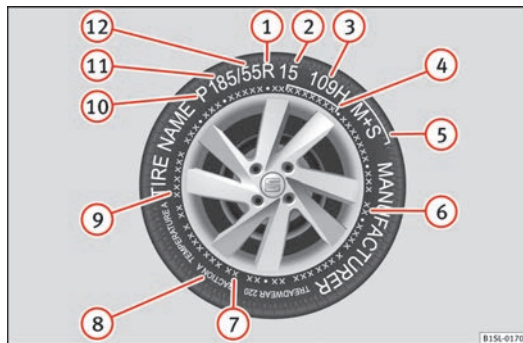
Abb. 127 Internationale Reifenbeschriftung.
