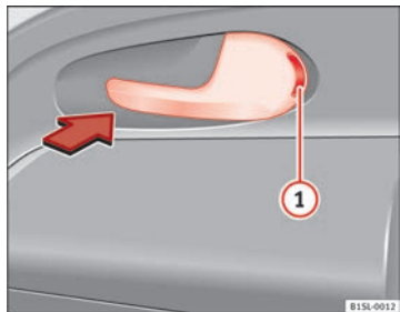
Abb. 20 In der Beifahrertür: Türöffnungshebel zum mechanischen Verriegeln.
