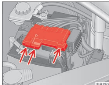
Abb. 118 Im Motorraum: Abdeckung für die Fahrzeugbatterie abnehmen.
