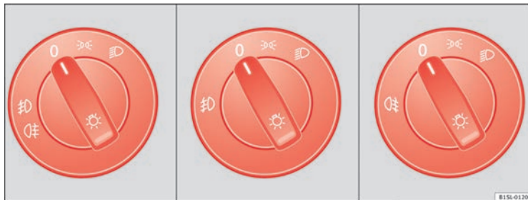
Abb. 56 Neben dem Lenkrad: Darstellung einiger Varianten des Lichtschalters.
