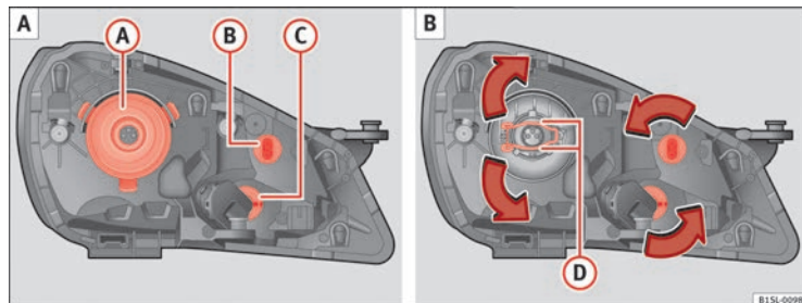
Abb. 153 Im Motorraum: Rückansicht des linken Frontscheinwerfers mit Gummiabdeckung: (A) Abblendlicht und Fernlicht, (B) Standlicht und Tagfahrlicht, (C) Blinklicht.
