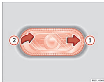
Abb. 160 Seitliche Blinkleuchte ausbauen.
