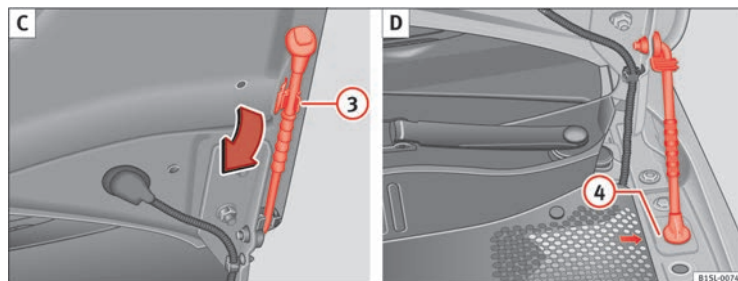
Abb. 113 C: Klappenstütze an der Motorraumklappe. D: Mit der Klappenstütze gesicherte Motorraumklappe. ►
