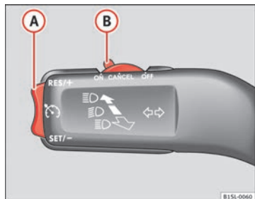
Abb. 98 Blinker- und Fernlichthebel links an der Lenksäule: Tasten und Schalter der GRA.
