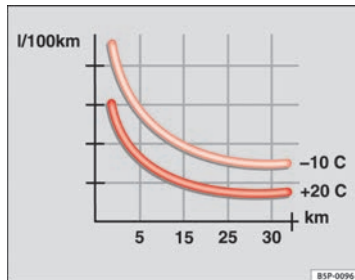
Abb. 95 Kraftstoffverbrauch in l/100 km bei 2 verschiedenen Umgebungstemperaturen.
