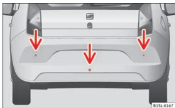
Abb. 96 Sensoren der Parkdistanzkontrolle im hinteren Stoßfänger.
