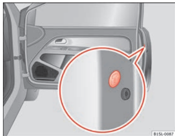
Abb. 136 In der Stirnseite der Beifahrertür: Notverriegelung, durch eine Gummichtung abgedeckt.
