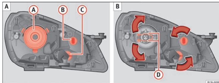
Abb. 150 Im Motorraum: Rückansicht des linken Frontscheinwerfers mit Gummiabdeckung: (A) Abblendlicht und Fernlicht, (B) Standlicht und Tagfahrlicht, (C) Blinklicht.
