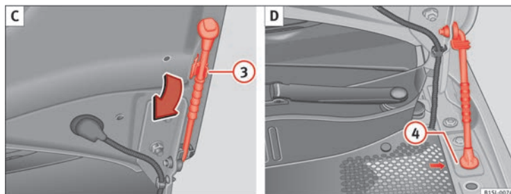
Abb. 110 C: Klappenstütze an der Motorraumklappe. D: Mit der Klappenstütze gesicherte Motorraumklappe. ►
