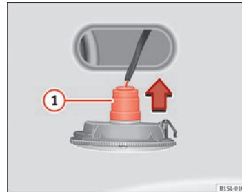
Abb. 158 Seitliche Blinkleuchte: Glühlampe auswechseln.
