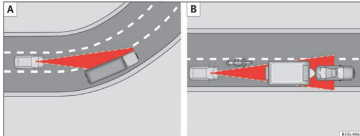
Abb. 99 A: Fahrzeug im Bereich einer Kurve. B: Vorausfahrender Motorradfahrer außerhalb des Wirkungsbereichs des Lasersensors.
