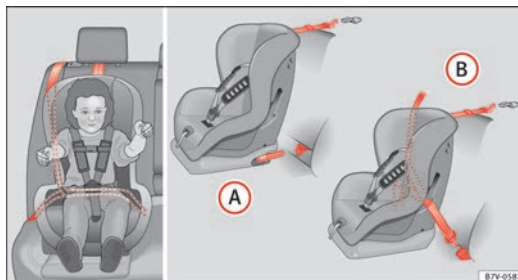
Abb. 52 Auf den Rücksitzen: Abbildung (A) zeigt die prinzipielle Befestigung des Kinderrückhaltesystems an den unteren Halteösen und mit oberem Befestigungsgurt. Abbildung (B) zeigt die Befestigung des Kinderrückhaltesystems mit dem Sicherheitsgurt des Fahrzeugs.
