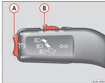
Abb. 95 Blinker- und Fernlichthebel links an der Lenksäule: Tasten und Schalter der GRA.
