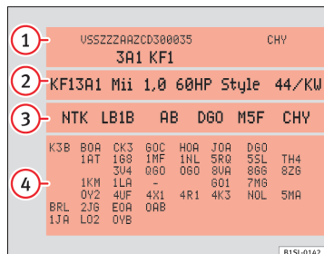
Abb. 163 A: Fahrzeugdatenträger; im Beispielbild mit Motorkennbuchstabe CBFA ③. B: Typschild.
