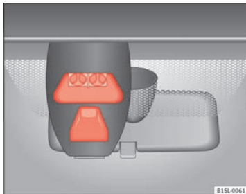
Abb. 96 An der Frontscheibe: Lasersensor für den City-Safety-Assistent.
