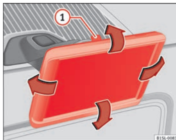
Abb. 125 In der Mittelkonsole: Navigationsgerät ausbauen.
