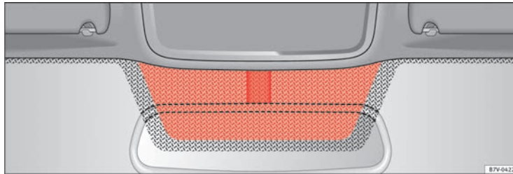
Abb. 59 Metallbeschichtete Infrarot-Frontscheibe mit Kommunikationsfenster (rote Fläche).
