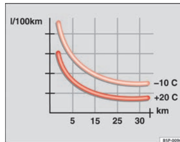
Abb. 92 Kraftstoffverbrauch in l/100 km bei 2 verschiedenen Umgebungstemperaturen.
