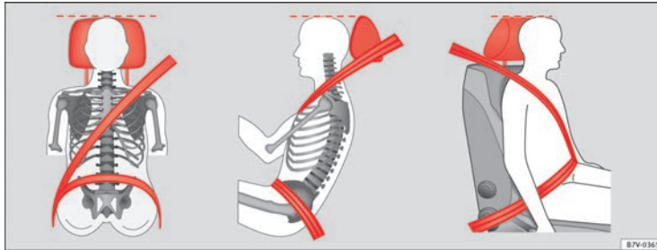
Abb. 44 Richtiges Gurtbandverlauf.
