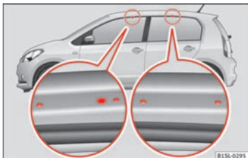
Abb. 142 Befestigungspunkte für Grundträger und Dachgepäckträger in 4-türigen Fahrzeugen.
