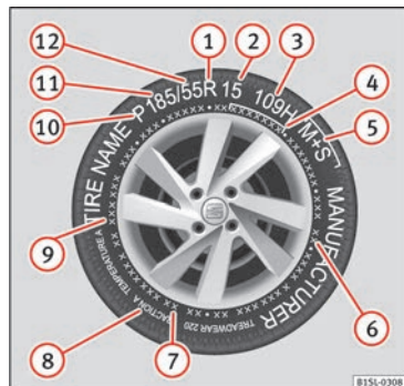
Abb. 178 Internationale Reifenbeschriftung.
