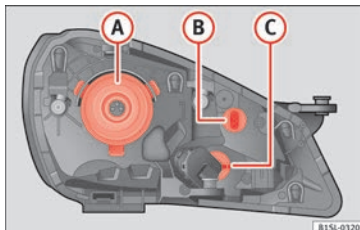
Abb. 84 Im Motorraum: Rückansicht des linken Scheinwerfers mit Gummiabdeckung: A Abblendlicht und Fernlicht, B Standlicht und Tagfahrlicht, C Blinker.
