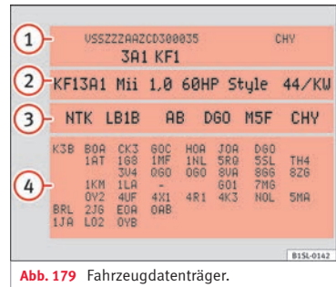
Abb. 179 Fahrzeugdatenträger.
