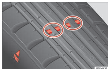
Abb. 175 Reifenprofil: Verschleißanzeiger.
