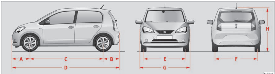
Abb. 181 Abmessungen
