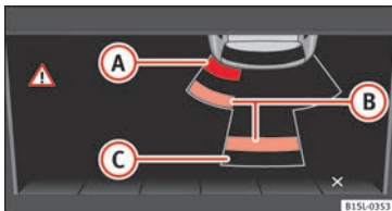
Abb. 152 Anzeige im Display des OPS: A Hindernis im Kollisionsbereich erkannt; B Hindernis im Segment erkannt; C abgetasteter Bereich hinter dem Fahrzeug.
