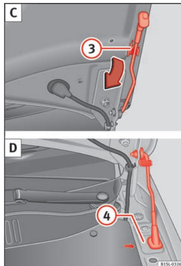
Abb. 9 C: Klappenstütze an der Motorraumklappe. D: Mit der Klappenstütze gesicherte Motorraumklappe.
