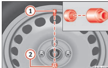
Abb. 54 Radwechsel: Reifenventil ① und Ort der Anti-Diebstahl-Radschraube ②.
