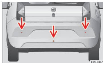
Abb. 151 Sensoren der Parkdistanzkontrolle im hinteren Stoßfänger.
