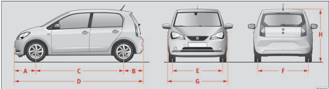
Abb. 181 Abmessungen
