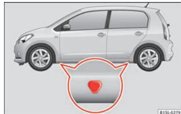
Abb. 55 Aufnahmeplätze für den Wagenheber.
