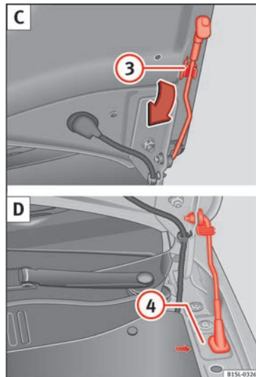
Abb. 9 C: Klappenstütze an der Motorraumklappe. C: Mit der Klappenstütze gesicherte Motorraumklappe.
