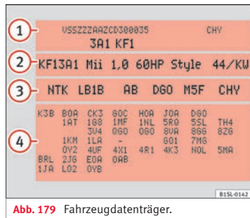
Abb. 179 Fahrzeugdatenträger.
