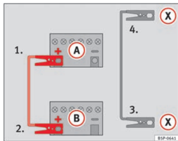
Abb. 181 Schaltschema zum Anschluss der Starthilfekabel, falls das stromgebende Fahrzeug mit einem Start-Stopp-System ausgestattet ist: entladene Batterie (A) und stromgebende Batterie (B).
