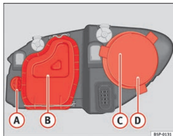
Abb. 162 Glühlampen des Hauptscheinwerfers
