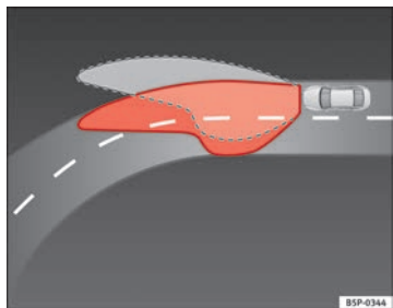
Abb. 74 Beleuchtung der Kurve mit Kurvenfahrlicht
