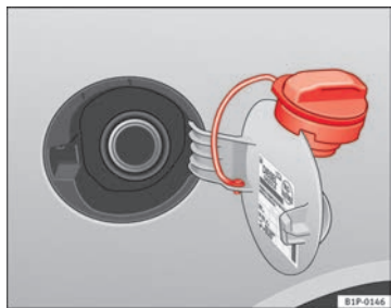
Abb. 138 Geöffnete Tankklappe
