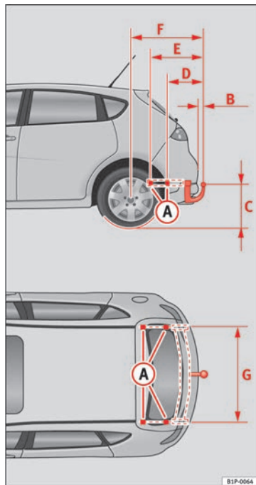
Abb. 137 Befestigungspunkte für die Anhängervorrichtung
