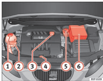
Abb. 185 Abbildung für die Einbaustellen der Elemente
