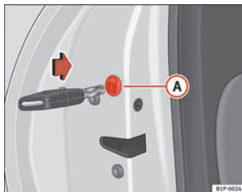
Abb. 59 Notverriegelung der Türen
