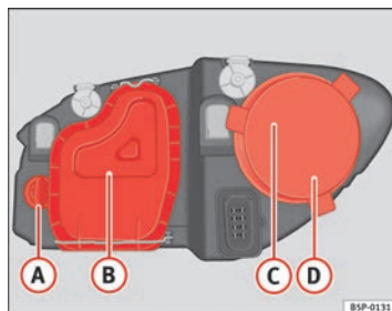
Abb. 164 Glühlampen des Hauptscheinwerfers ▶
