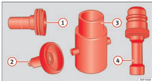
Abb. 141 Übersicht der Adapter für den LPG-Einfüllstutzen.
