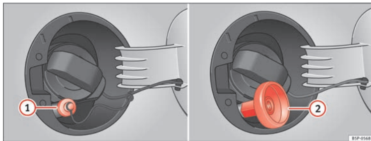
Abb. 139 Geöffneter Tankdeckel mit Autogas-Einfüllstutzen und Adapter.
