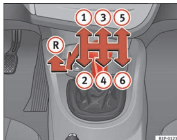
Abb. 123 In der Mittelkonsole: Schaltschema eines 6-Gang-Schaltgetriebes
