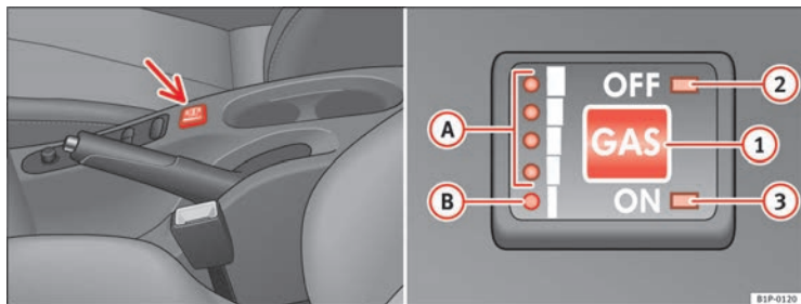
Abb. 35 Mittelkonsole: Schalter und Kontrollleuchten der Autogasanlage.
