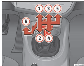
Abb. 122 In der Mittelkonsole: Schaltschema eines 5-Gang-Schaltgetriebes
