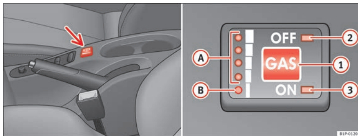
Abb. 119 Mittelkonsole: Schalter und Kontrollleuchten der Autogasanlage.
