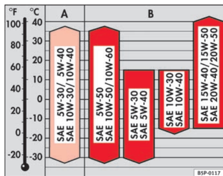
Abb. 138 Öltypen nach Temperaturbereichen
