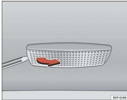
Abb. 174 Ausbau der Leuchte in der Sonnenblende
