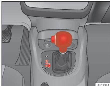
Abb. 123 Wählhebelsperre lösen
