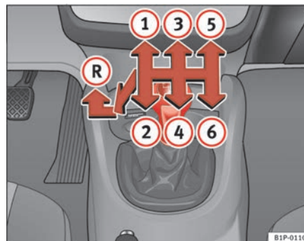
Abb. 120 In der Mittelkonsole: Schaltschema eines 6-Gang-Schaltgetriebes
