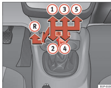
Abb. 119 In der Mittelkonsole: Schaltschema eines 5-Gang-Schaltgetriebes
