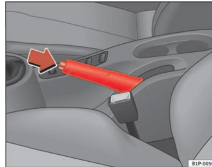
Abb. 124 Handbremse zwischen den Vordersitzen
