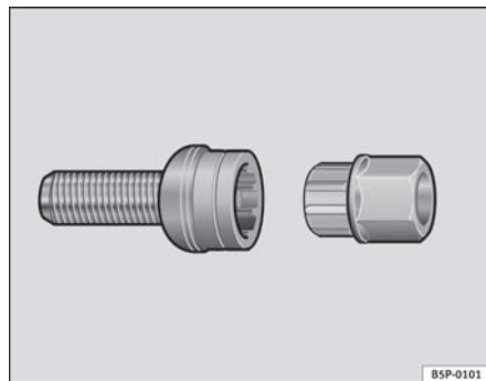
Abb. 159 Diebstahlhemmende Radschrauben
