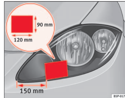
Abb. 133 Linker Scheinwerfer
