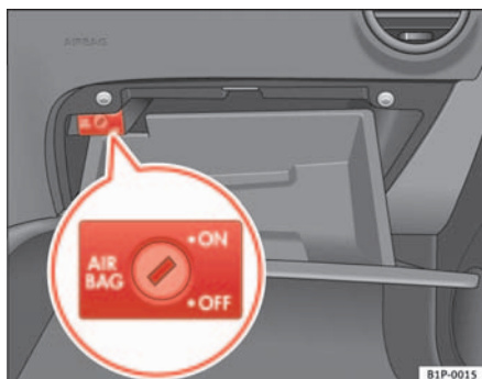
Abb. 25 Im Handschuhkasten: Schlüsselschalter zum Ab- und Einschalten der Airbags auf der Beifahrerseite
