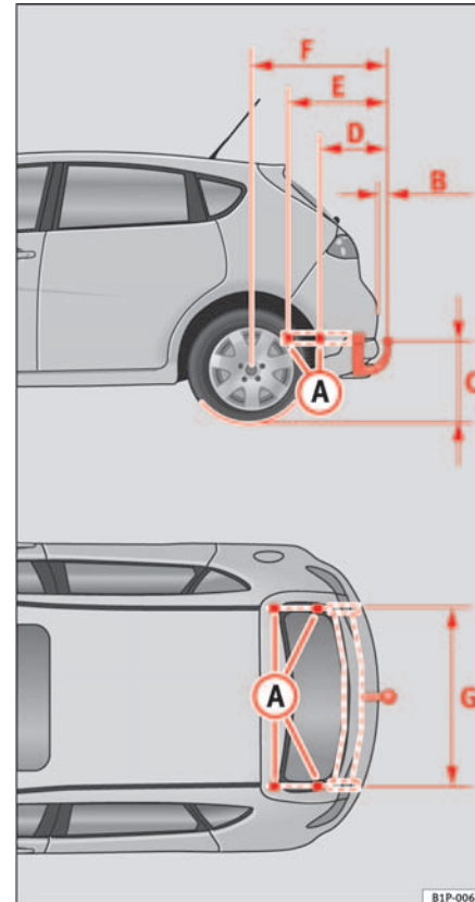
Abb. 139 Befestigungspunkte für die Anhängervorrichtung
