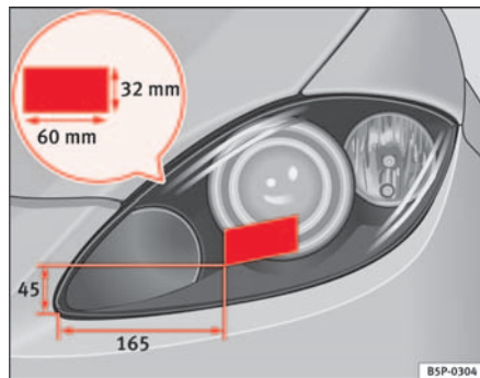
Abb. 137 Linker Scheinwerfer
