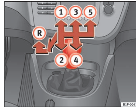
Abb. 116 Ausschnitt aus der Mittelkonsole: Schalt-schema vom 5-Gang-Schaltgetriebe
