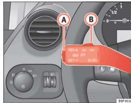
Abb. 129 Blinker- und Fernlichthebel: Schalter und Wippe für GRA
