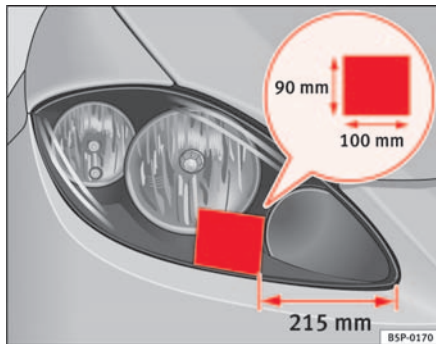
Abb. 132 Rechter Scheinwerfer
