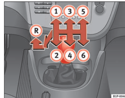
Abb. 117 Ausschnitt aus der Mittelkonsole: Schalt-schema vom 6-Gang-Schaltgetriebe
