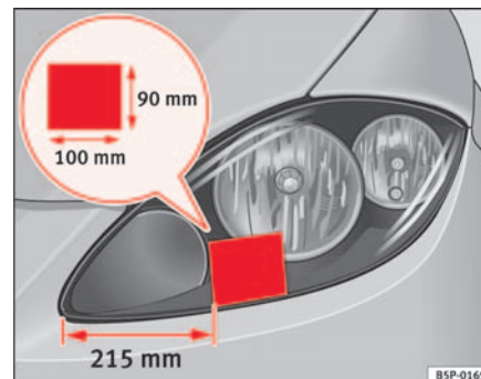
Abb. 131 Linker Scheinwerfer
