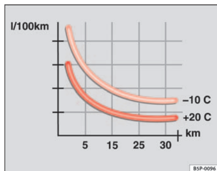
Abb. 138 Kraftstoffverbrauch in l/100km bei zwei verschiedenen Umgebungstemperaturen
