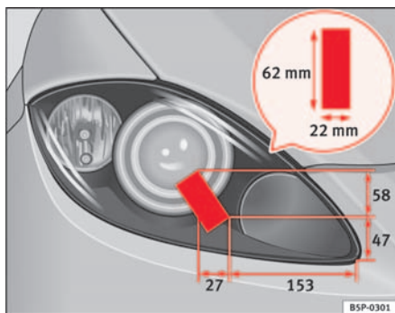
Abb. 134 Rechter Scheinwerfer
