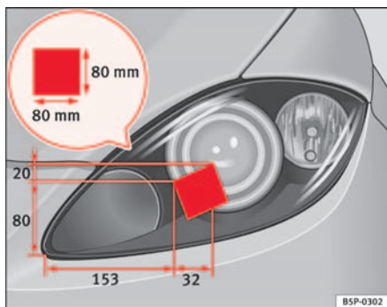
Abb. 135 Linker Scheinwerfer
