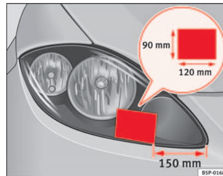
Abb. 130 Rechter Scheinwerfer
