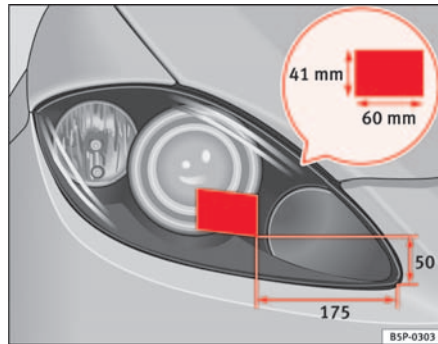
Abb. 136 Rechter Scheinwerfer
