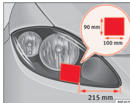
Abb. 129 Rechter Scheinwerfer
