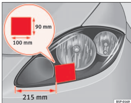
Abb. 128 Linker Scheinwerfer
