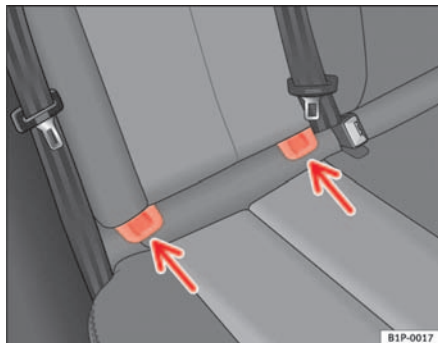
Abb. 30 ISOFIX-Halteösen
