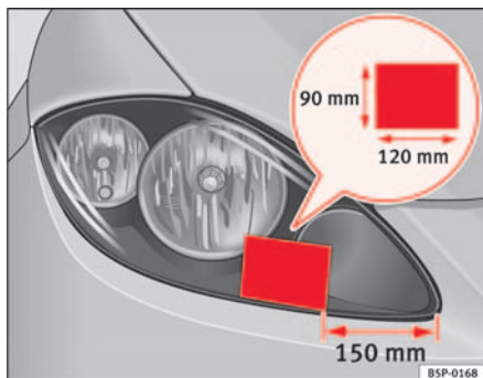
Abb. 127 Rechter Scheinwerfer
