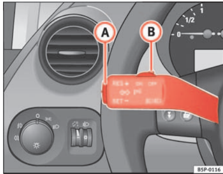
Abb. 126 Blinker- und Fernlichthebel: Schalter und Wippe für GRA
