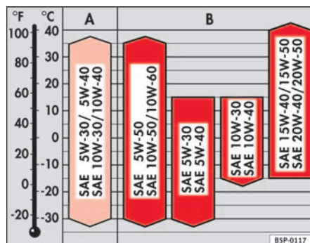
Abb. 136 Öltypen nach Temperaturbereichen
