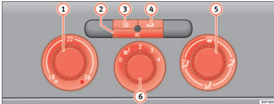
Abb. 107 In der Instrumententafel: Bedienelemente der Climatic
