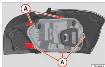
Abb. 119 Befestigungslaschen Rückseite Heckleuchte.
