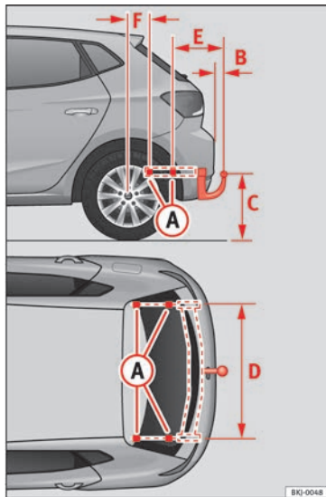
Abb. 226 Befestigungspunkte für die Anhängervorrichtung
