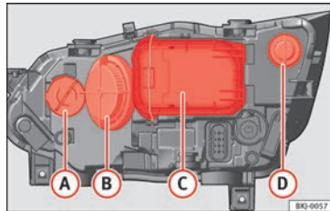
Abb. 112 Halogen-Hauptscheinwerfer
