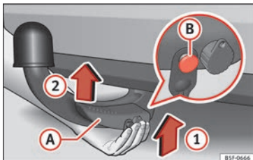
Abb. 217 Anbringen abnehmbaren Kugelkopf/Entriegelungsbolzen im entfalteten Zustand
