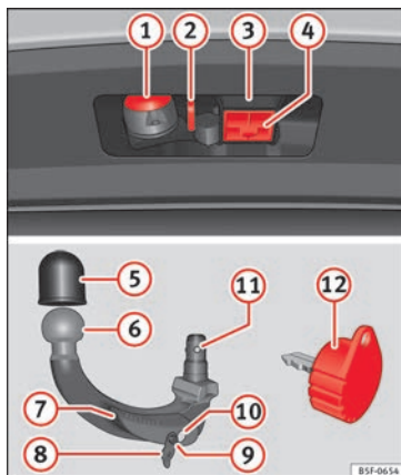
Abb. 213 Halterung der Anhängervorrichtung / abnehmbarer Kugelkopf / Schlüssel
