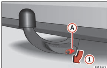
Abb. 221 Schließabdeckung abnehmen
