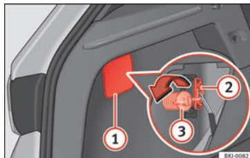
Abb. 118 Gepäckraum: Zugang zur Befestigungsschraube der Heckleuchte
