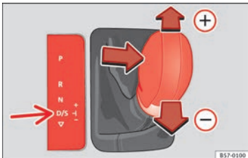
Abb. 183 Mittelkonsole: zu Tiptronic ändern.
