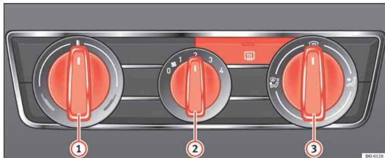
Abb. 174 Bedienelemente der Heizung in der Instrumententafel.
