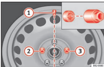
Abb. 84 Radwechsel: Reifenventil ① und Einbauort der Anti-Diebstahl-Radschraube ② oder ③.
