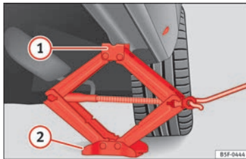
Abb. 86 Wagenheber anbringen
