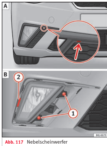
Abb. 117 Nebelscheinwerfer
