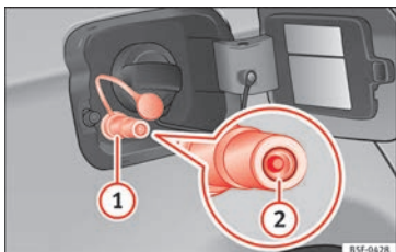
Abb. 227 Geöffnete Tankklappe: Gas-Einfüllstutzen ①, Dichting des Einfüllstutzens ②.
