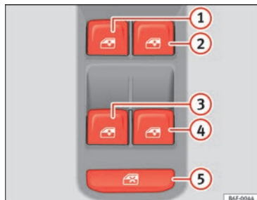
Abb. 146 Ausschnitt aus der Fahrertür: Bedienelemente für die vorderen und hinteren Fenster (Fahrzeug mit elektrischen Fensterhebern vorne und hinten).
