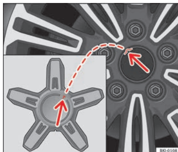
Abb. 80 Radvollblende anbringen
