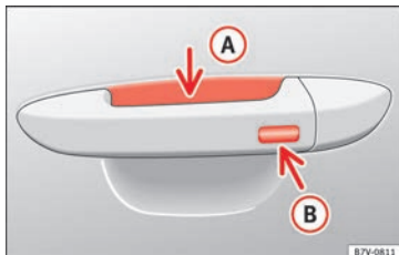
Abb. 144 Schlüsselloses Schließ- und Startsystem Keyless Access: Sensorfläche A zur Entriegelung auf der Innenseite des Türgriffs und Sensorfläche B zur Verriegelung auf der Außenseite des Türgriffs.
