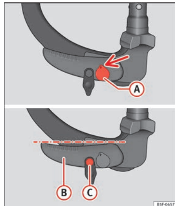
Abb. 216 Ruheposition: Stellung von Hebel und Entriegelungsbolzen
