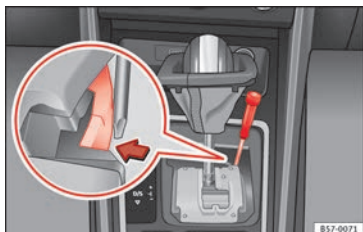
Abb. 60 Wählhebel: Notentriegeln aus der Parkstellung
