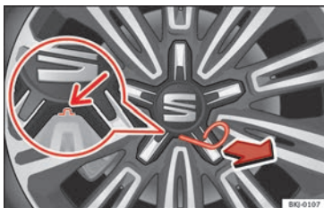
Abb. 79 Radvollblende abziehen
