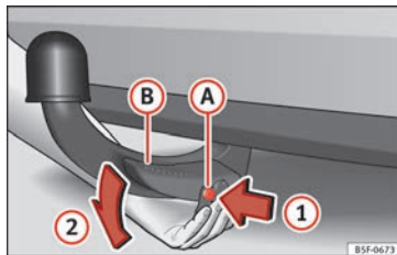
Abb. 223 Abnehmbaren Kugelkopf lösen
