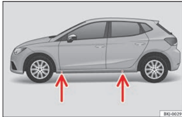
Abb. 85 Aufnahmepunkte für den Wagenheber.
