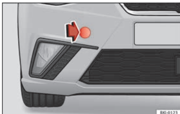
Abb. 108 Vorderer Stoßfänger, rechte Seite: Abdeckung abziehen.
