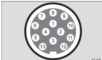
Abb. 224 Schematische Darstellung: Zuweisung der Steckverbinderstifte für Anhängerstrom.
