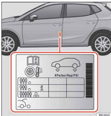
Abb. 231 Einbauort des Aufklebers für den Reifenfülldruck.
