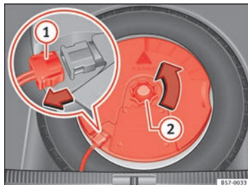
Abb. 235 Im Gepäckraum: Subwoofer ausbauen.
