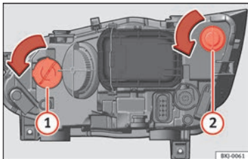
Abb. 116 Im Motorraum: Glühlampe Blinker 1 und Glühlampe Tagfahrlicht / Standlicht 2 .
