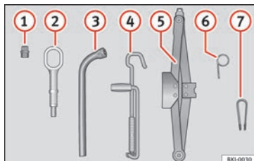
Abb. 77 Im Gepäckraum unter dem Gepäckraumboden: Bordwerkzeug.
