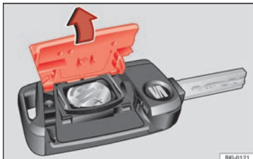
Abb. 138 Fahrzeugschlüssel: Deckel des Batterie-fachs öffnen.
