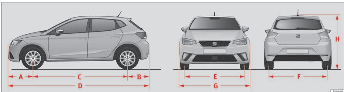
Abb. 238 Abmessungen
