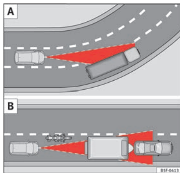
Abb. 201 (A) Fahrzeug in einer Kurve. (B) Vorausfahrender Motorradfahrer außerhalb des Erfassungsbereichs des Radarsensors.
