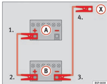
Abb. 168 Anschluss-schemata für Fahrzeuge ohne Start-Stopp-System.
