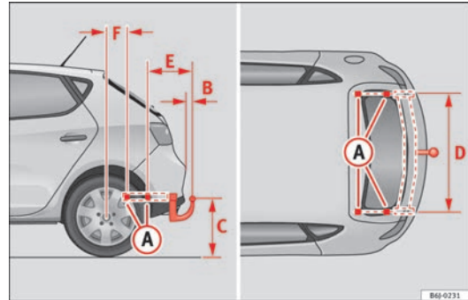
Abb. 118 Befestigungspunkte für die Anhängavorrichtung
