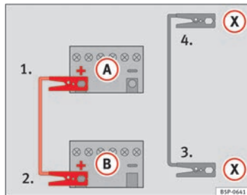
Abb. 169 Anschluss-schemata für Fahrzeuge mit Start-Stopp-System.
