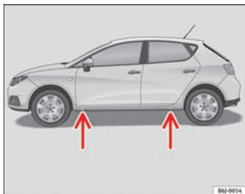
Abb. 138 Aufnahme- punkte für den Wagen- heber
