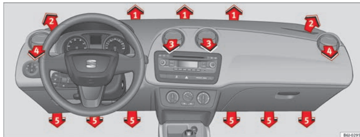
Abb. 93 Luftaustrittsdüsen ▶
