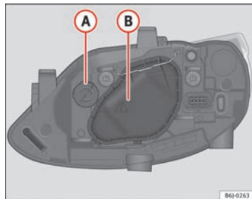
Abb. 156 Glühlampen des AFS-Scheinwerfers
