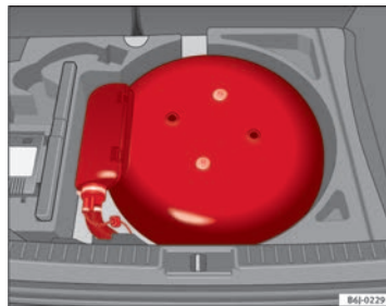
Abb. 121 Autogas-Vorratsbehälter in der Reservardmulde.
