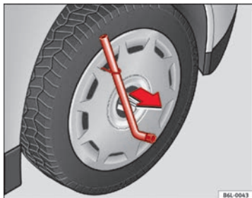
Abb. 136 Die Radvollblende vom Rad abnehmen
