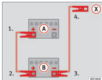
Abb. 168 Schaltschema zum Anschluss der Starthilfekabel, falls das stromgebende Fahrzeug über kein Start-Stopp-System verfügt: entladene Batterie (A) und stromgebende Batterie (B).
