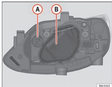
Abb. 156 Glühlampen des AFS-Scheinwerfers
