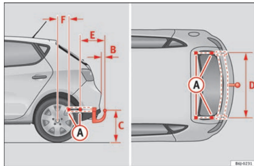
Abb. 118 Befestigungspunkte für die Anhängervorrichtung
