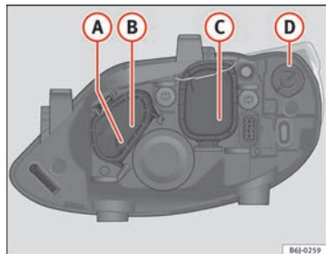
Abb. 148 Doppelscheinwerfer
