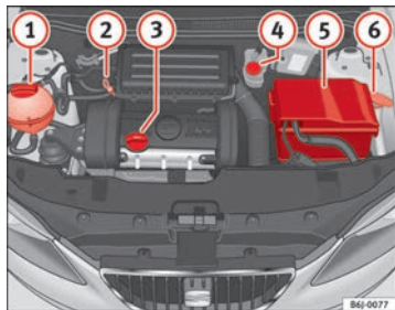
Abb. 173 Abbildung für die Einbaustellen der Elemente
