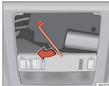
Abb. 53 Notbetätigung Panoramadach / Ausstelldach
