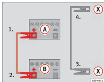
Abb. 169 Schaltschema zum Anschluss der Starthilfekabel, falls das stromgebende Fahrzeug mit einem Start-Stopp-System ausgestattet ist: entladene Batterie (A) und stromgebende Batterie (B).
