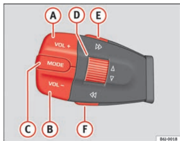
Abb. 41 Schalter Audio-Steuerung
