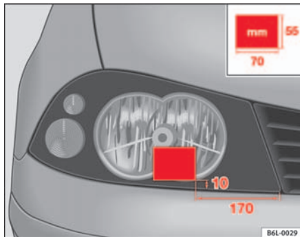
Abb. 112 Rechter Scheinwerfer
