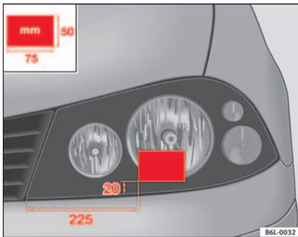
Abb. 115 Linker Schein- werfer
