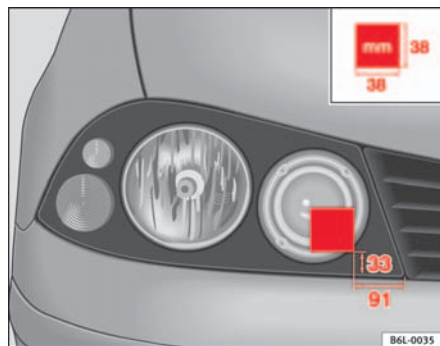
Abb. 118 Rechter Scheinwerfer
