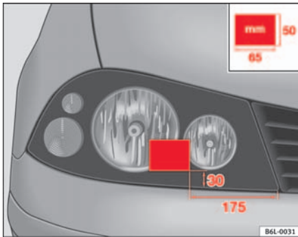
Abb. 114 Rechter Scheinwerfer
