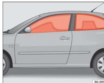
Abb. 23 Aufgeblasene Kopfairbags
