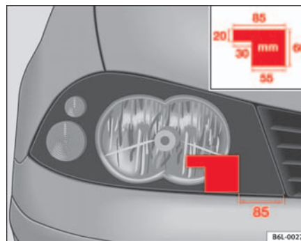
Abb. 110 Rechter Scheinwerfer
