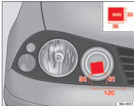
Abb. 120 Rechter Scheinwerfer
