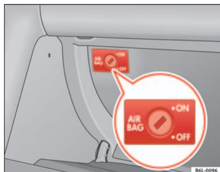
Abb. 24 Im Handschuhfach: Schlüsselschalter zum Ab- und Einschalten der Airbags auf der Beifahrerseite
