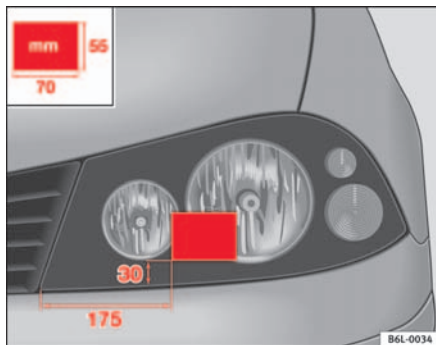
Abb. 117 Linker Scheinwerfer
