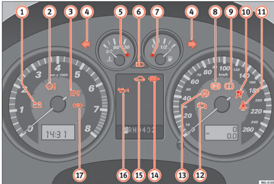
Abb. 39 Kombiinstrument mit Warn- und Kontrollleuchten. Einige der hier aufgeführten Warn- und Kontrollleuchten gehören zu bestimmten Modellausführungen oder sind Bestandteil von Mehrausstattungen ▶
