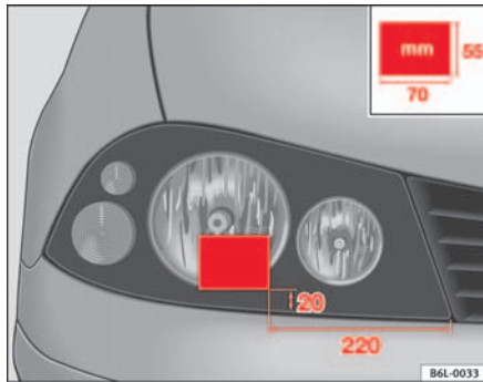
Abb. 116 Rechter Scheinwerfer
