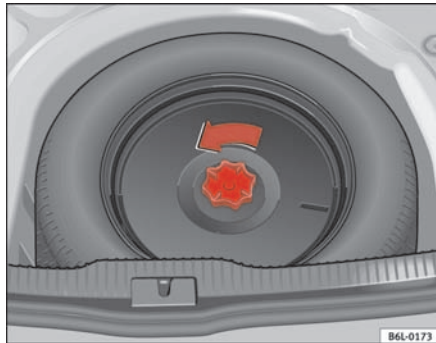
Abb. 137 Zugang zum Reserverad
