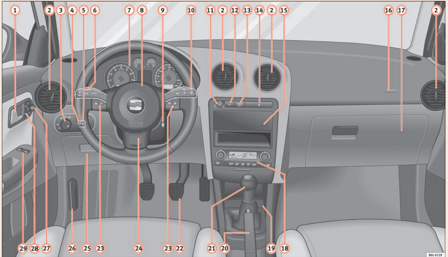
Abb. 30 Instrumententafel
