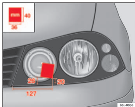
Abb. 119 Linker Schein- werfer
