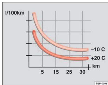
Abb. 122 Kraftstoffverbrauch in l/100km bei zwei verschiedenen Umgebungstemperaturen
