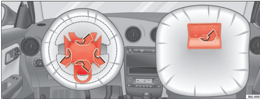
Abb. 19 Airbagabdeckungen bei ausgelösten Frontairbags
