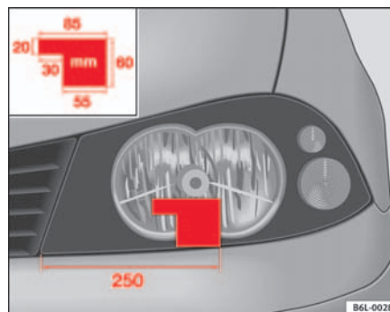
Abb. 111 Linker Scheinwerfer
