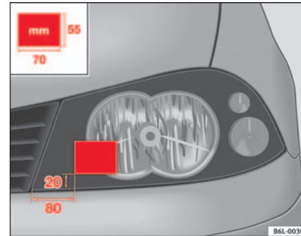
Abb. 113 Linker Scheinwerfer
