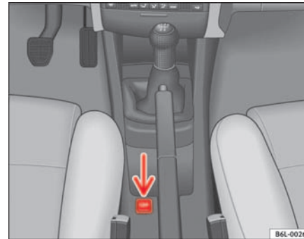
Abb. 98 Ausschnitt aus der Mittelkonsole: ESP-Taste
