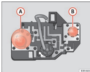
Abb. 233 Position der Glühlampen am Lampenträger. Beispiel: Heckleuchte in der Heckklappe
