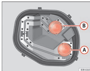
Abb. 223 Position der Glühlampen am Lampenträger: Beispiel: linke äußere Heckleuchte.
