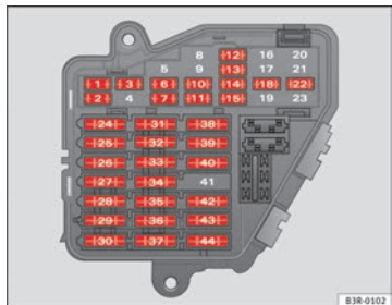
Abb. 200 Prinzipdarstellung des Sicherungsträgers an der linken Stirnseite der Instrumententafel: Sicherungen (ohne Sicherungsdeckel)
