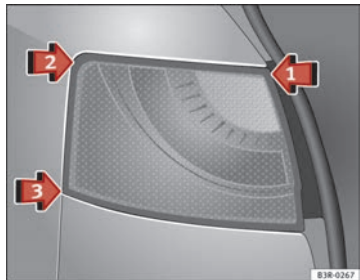
Abb. 226 Heckleuchte einbauen
