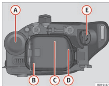
Abb. 203 Glühlampen des Halogenscheinwerfers
