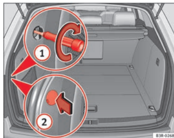
Abb. 227 Gepäckraum: Lage der Befestigungsschraube für Heckleuchte
