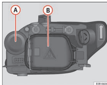
Abb. 215 Glühlampen für Bi-Xenon-Scheinwerfer AFS
