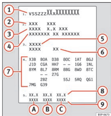
Abb. 243 Fahrzeugdatenträger (Gepäckraum)
