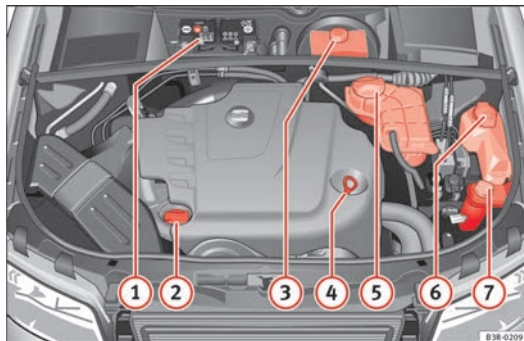
Abb. 244 Abbildung für die Einbaustellen der Elemente
