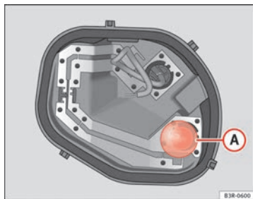
Abb. 224 Position der Glühlampen am Lampenträger: Beispiel: linke äußere Heckleuchte.
