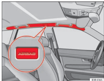
Abb. 25 Einbaulage der Kopfairbags auf der linken Fahrzeugseite
