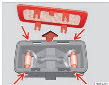
Abb. 236 Gepäckraum- beleuchtung
