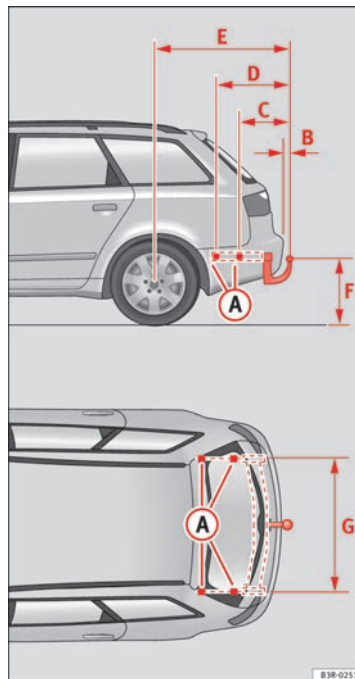
Abb. 172 Befestigungspunkte für die Anhangevorrichtung
