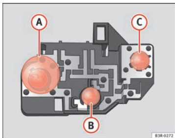
Abb. 232 Position der Glühlampen am Lampenträger. Beispiel: Heckleuchte in der Heckklappe
