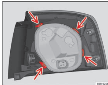
Abb. 225 Befestigen Sie den Lampenträger an der Heckleuchte
