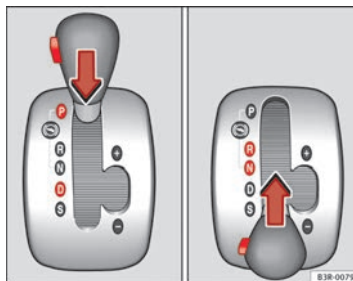
Abb. 149 Wählhebelsperre
