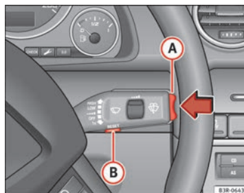
Abb. 61 Scheibenwischerhebel: Bedienelemente des Bordcomputers
