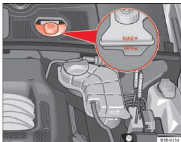
Abb. 176 Motorraum: Markierungen am Bremsflüssigkeitsbehälter
