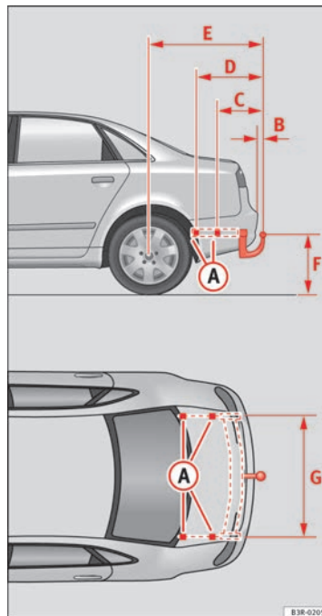
Abb. 165 Befestigungspunkte für die Anhangevorrichtung
