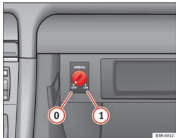
Abb. 28 Im Handschuhfach: Schüsselschalter zum Ein- und Abschalten des Beifahrer-Airbags
