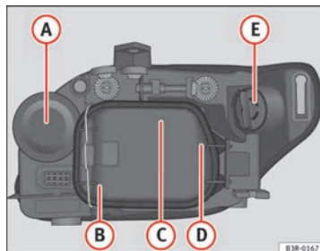
Abb. 193 Glühlampen des Halogenscheinwerfers
