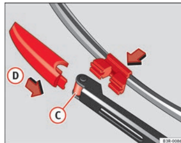
Abb. 175 Wischerblatt befestigen
