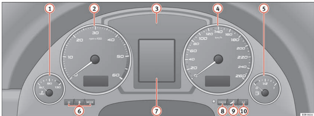
Abb. 38 Übersicht Kombiinstrument
