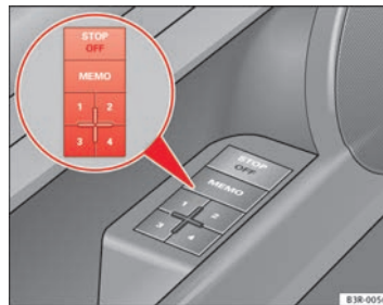
Abb. 109 Fahrertür: Memory-System
