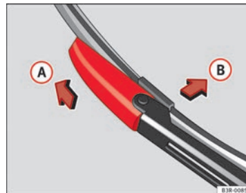
Abb. 174 Wischerblatt abnehmen
