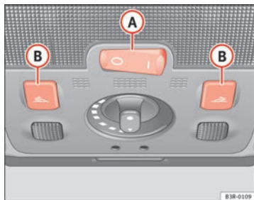
Abb. 92 Ausschnitt aus Dachhimmel: Innenbeleuchtung vorne
