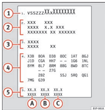
Abb. 233 Fahrzeugdatenträger (Gepäckraum)
