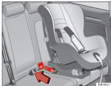
Abb. 34 Die ISOFIX-Rastarme des Kindersitzes lassen sich über die bereits angebrachten Plastikführungen einführen, bis sie in den ISOFIX-Verankerungen des Fahrzeugs einrasten.
