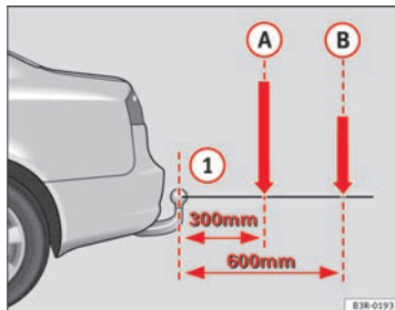
Abb. 154 Prinzipdarstellung der Lastverteilung von Anbauteilen und Zubehör
