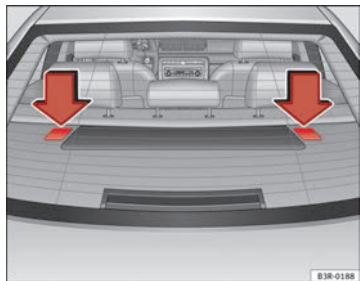
Abb. 35 Lage der Top Tether-Ösen an der hinteren Ablage
