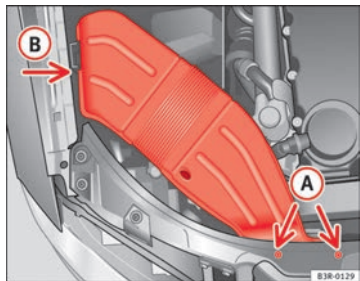
Abb. 204 Luftführungshutze an rechter Fahrzeugseite
