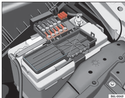
Abb. 137 Sicherungs- kasten auf Batterie
