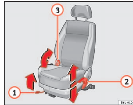
Abb. 71 Bedienelemente am linken Vordersitz
