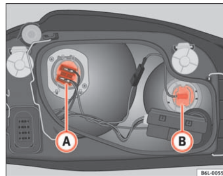
Abb. 138 Glühlampe des Hauptscheinwerfers
