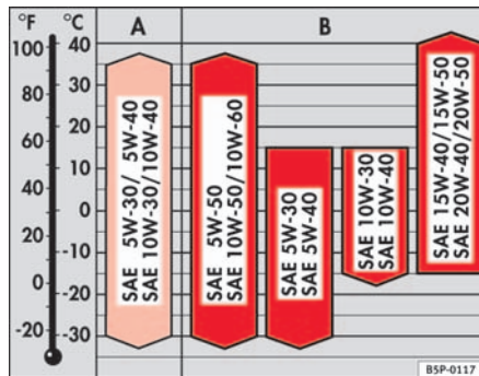
Abb. 119 Öltypen nach Temperaturbereichen
