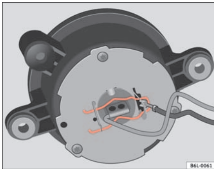
Abb. 149 Nebelscheinwerfer
