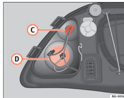
Abb. 139 Glühlampe des Hauptscheinwerfers
