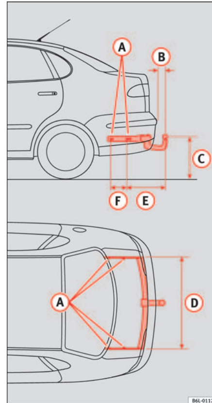
Abb. 116 Befestigungspunkte für die Anhangvorrichtung
