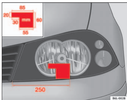
Abb. 104 Linker Scheinwerfer
