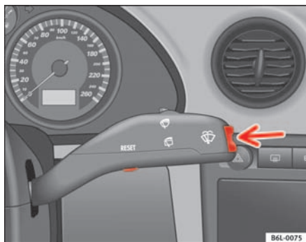
Abb. 35 Scheinwischer- und Scheibenwascherhebel: Taste A und Wippe B
