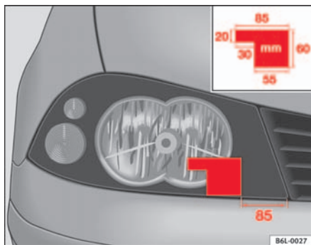
Abb. 103 Rechter Scheinwerfer
