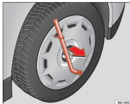
Abb. 130 Die Radvoll- blende vom Rad abnehmen.
