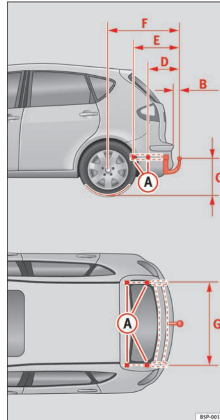
Abb. 158 Befestigungspunkte für die Anhangervorrichtung
