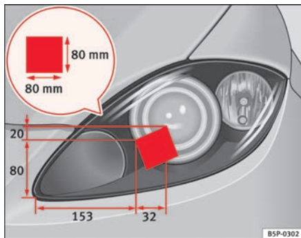
Abb. 155 Linker Scheinwerfer
