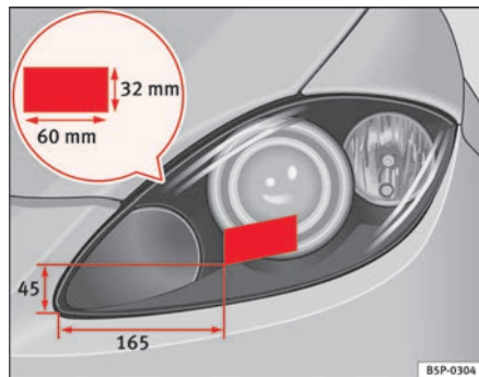
Abb. 157 Linker Scheinwerfer
