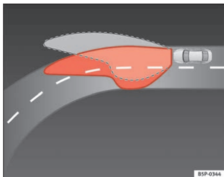
Abb. 76 Beleuchtung der Kurve mit automatisch gerichteten Scheinwerfern
