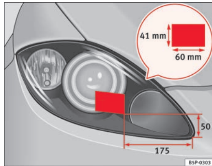
Abb. 156 Rechter Scheinwerfer
