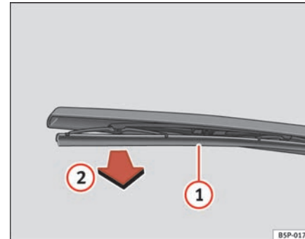
Abb. 169 Scheibenwischerblatt hinten auswechseln
