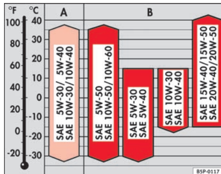
Abb. 162 Öltypen nach Temperaturbereichen
