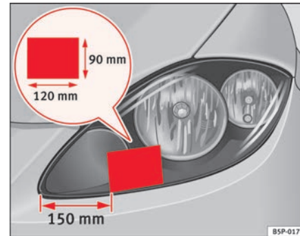
Abb. 153 Linker Scheinwerfer
