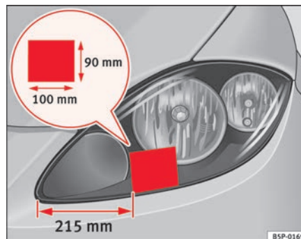
Abb. 151 Linker Scheinwerfer
