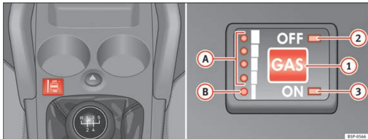
Abb. 36 Mittelkonsole: Schalter und Kontrollleuchten der Autogasanlage.
