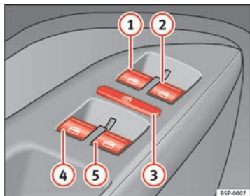
Abb. 69 Ausschnitt aus der Fahrertür: Schalter für die Fenster vorne und hinten
