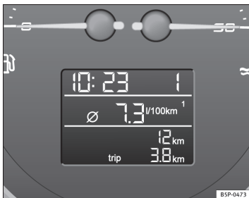
Abb. 41 Display im Kombiinstrument
