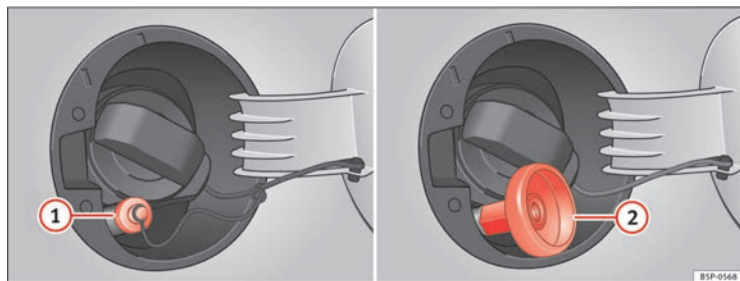
Abb. 158 Geöffneter Tankdeckel mit Autogas-Einfüllstutzen und Adapter.
