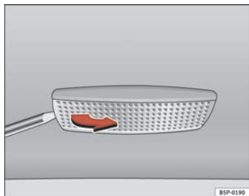
Abb. 202 Ausbau der Leuchte in der Sonnenblende
