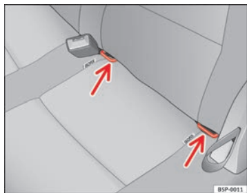
Abb. 31 ISOFIX-Halteösen
