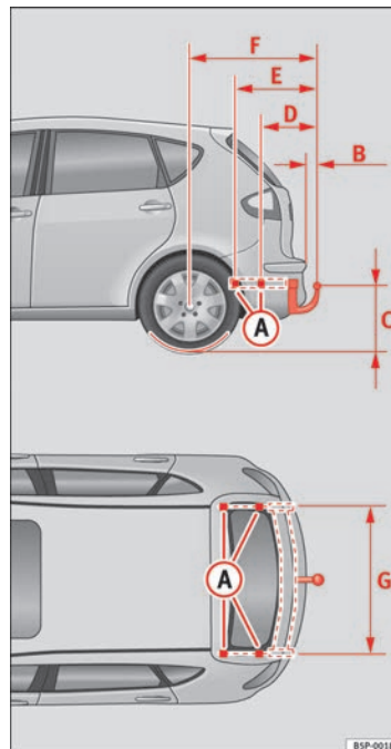
Abb. 156 Befestigungspunkte für die Anhangervorrichtung
