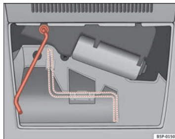
Abb. 72 Kurbel für Notverriegelung
