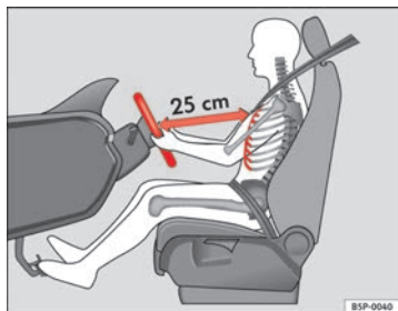
Abb. 1 Der richtige Abstand des Fahrers vom Lenkrad
