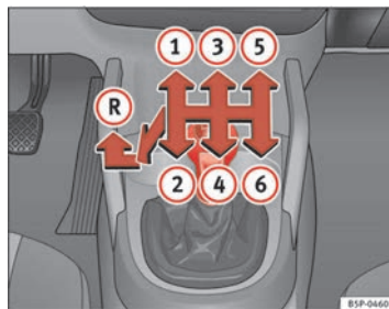
Abb. 142 In der Mittelkonsole: Schaltschema eines 6-Gang-Schaltgetriebes
