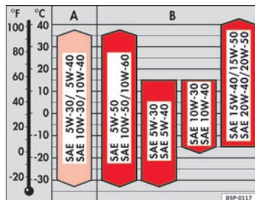
Abb. 163 Öltypen nach Temperaturbereichen
