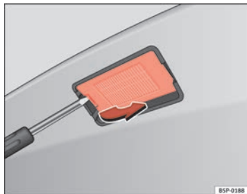
Abb. 200 Kennzeichenbeleuchtung
