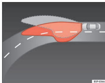
Abb. 76 Beleuchtung der Kurve mit automatisch gerichteten Scheinwerfern
