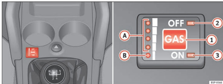
Abb. 138 Mittelkonsole: Schalter und Kontrollleuchten der Autogasanlage.
