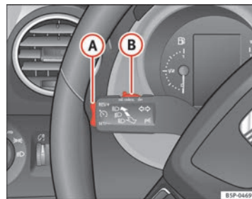
Abb. 155 Blinker- und Fernlichthebel: Schalter und Wippe für die Geschwindigkeitsregelanlage
