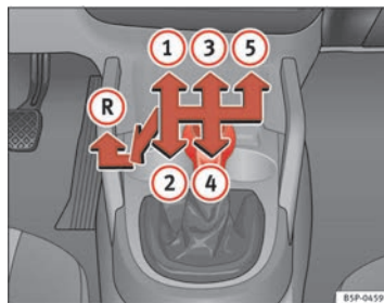
Abb. 141 In der Mittelkonsole: Schaltschema eines 5-Gang-Schaltgetriebes
