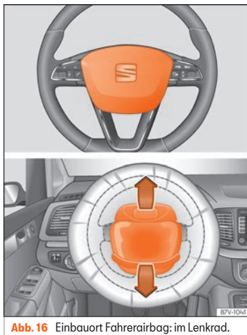
Abb. 16 Einbauort Fahrersairbag: im Lenkrad.
