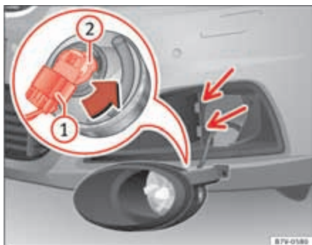
Abb. 205 Glühlampe im Scheinwerfer auswechseln.
