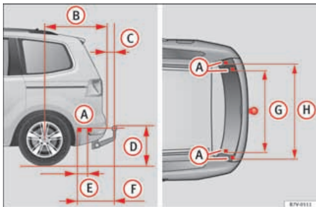
Abb. 154 Maße und Befestigungspunkte zum Nachrüsten einer Anhängervorrichtung.
