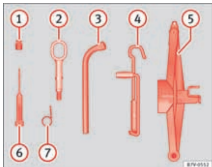
Abb. 195 Bestandteile des Bordwerkzeugs.
