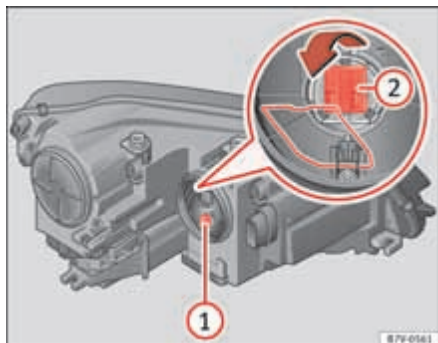
Abb. 203 Blinklichtlampenhalter (1) und Abbiegelicht (2).
