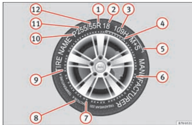
Abb. 175 Internationale Reifenbeschriftung.
