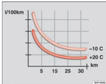
Abb. 152 Kraftstoffverbrauch in l/100 km bei zwei verschiedenen Umgebungstemperaturen.
