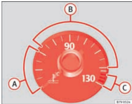
Abb. 167 Motorkühlmitteltemperaturanzeige im Kombiinstrument: A Kaltbereich; B Normalbereich; C Warnbereich.
