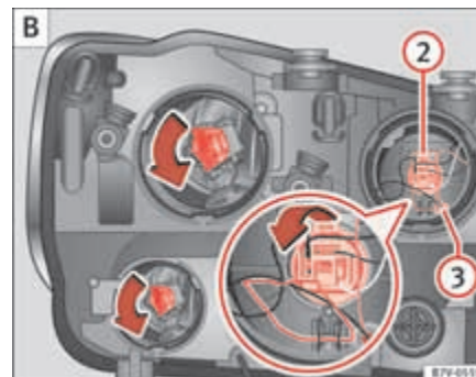
Abb. 201 Linker Scheinwerfer
