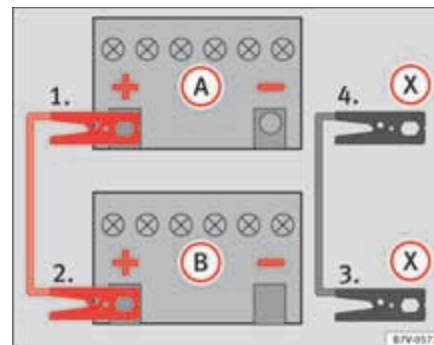
Abb. 214 Schema für das Anklemmen der Starthilfekabel bei Starthelferfahrzeugen mit Start-Stopp-Betrieb: entladene Fahrzeugbatterie (A) und Strom gebende Fahrzeugbatterie (B).
