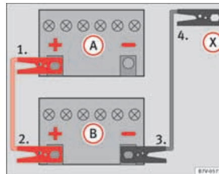
Abb. 213 Schema für das Anklemmen der Starthilfekabel bei Starthelferfahrzeugen ohne Start-Stopp-Betrieb: entladene Fahrzeugbatterie (A) und Strom gebende Fahrzeugbatterie (B).
