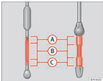
Abb. 165 Ölmesstab mit Motorölstandsmarkierungen.
