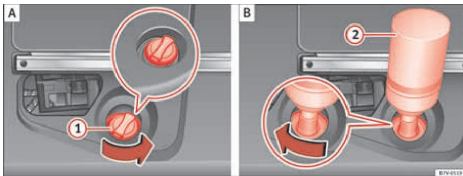
Abb. 162 AdBlue-Tank mit Verschluss des Tankeinfüllstutzens und Nachfüllflasche.
