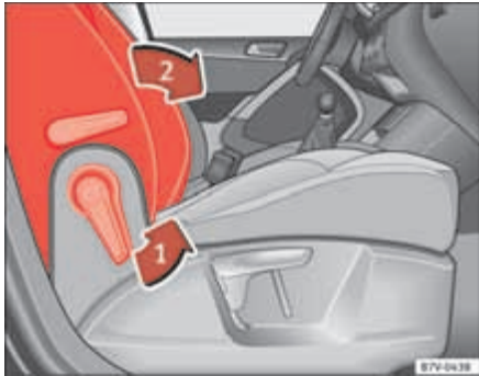
Abb. 82 Beifahrersitzlehne vorklappen.
