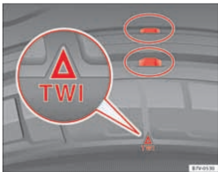
Abb. 174 Reifenprofil: Verschleißanzeiger.
