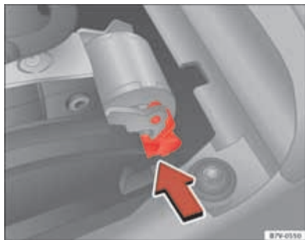
Abb. 193 Wählhebelsperre notentriegeln.
