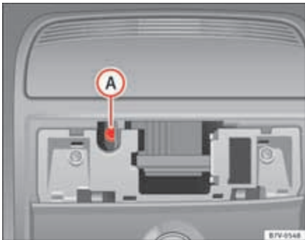
Abb. 191 Innensechskantschraube zum Schließen des Panorama-Schiebedachs.
