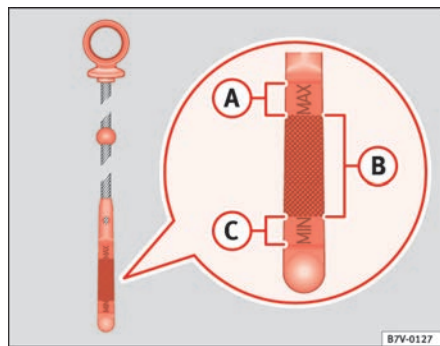
Abb. 141 Ölmesstab
