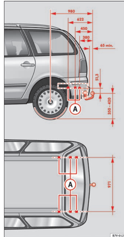
Abb. 136 Befestigungspunkte für die Anhangsvorrichtung
