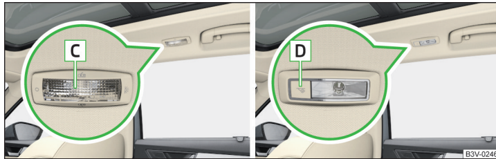
Abb. 73 Innenleuchte hinten: Variante 2 / Variante 3
