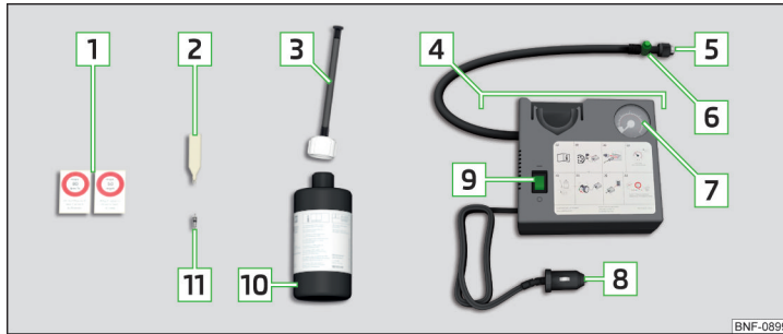
Abb. 335 Pannensetbeschreibung
