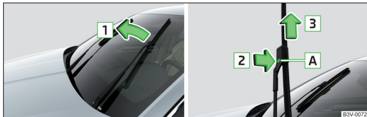
Abb. 351 Scheibenwischerblatt der Frontscheibe auswechseln
