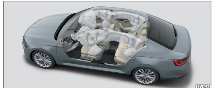
Abb. 20 Gasgefüllte Airbags
