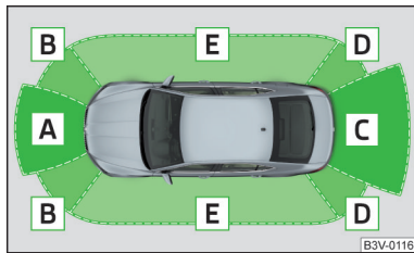
Abb. 269 Abgetastete Bereiche und Reichweite der Sensoren
