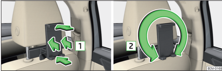
Abb. 136 Halter kippen und drehen
