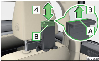
Abb. 137 Haltergröße anpassen
