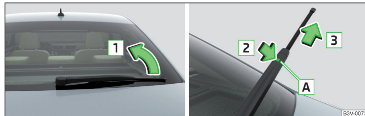
Abb. 352 Scheibenwischerblatt der Heckscheibe auswechseln
