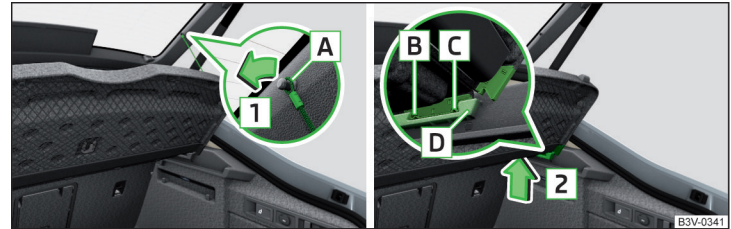
Abb. 144 Gepäckraumabdeckung herausnehmen
