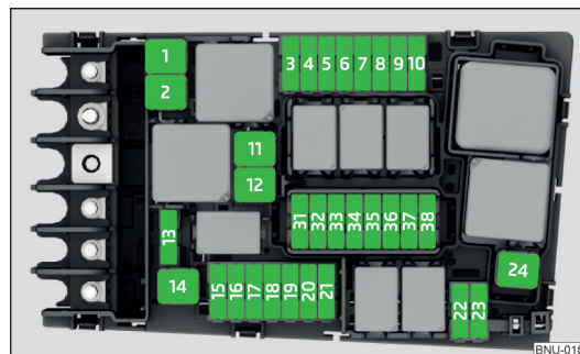
Abb. 359 Sicherungen
