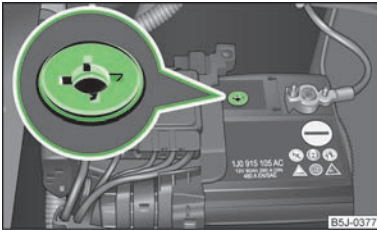
Abb. 121 Fahrzeugbatterie: Säurestandsanzeige
