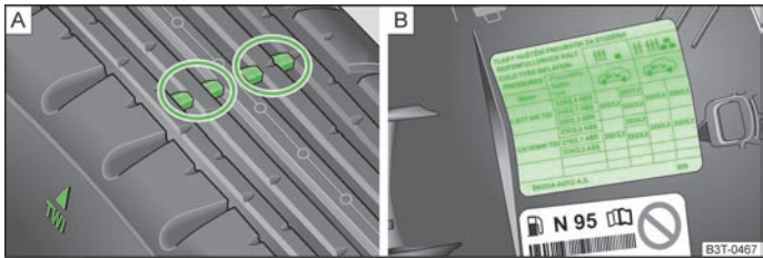
Abb. 122 Reifenprofil mit Verschleißanzeigern / Geöffnete Tankklappe mit einer Tabelle der Reifengrößen und -fülldruckwerte
