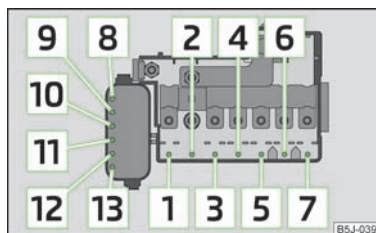
Abb. 141 Fahrzeugbatterie: Abdeckung des Sicherungskastens
