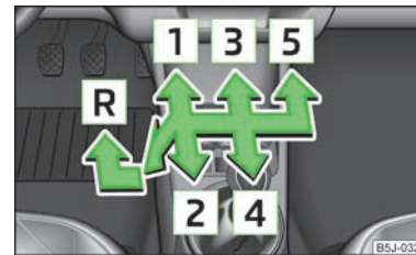
Abb. 79 Schaltschema des 5-Gang-Schaltgetriebes
