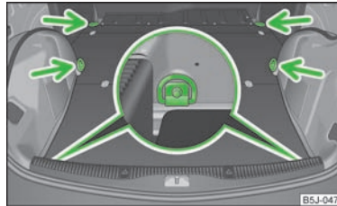
Abb. 154 Laderaum: Verzurrösen
