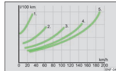
Abb. 108 Kraftstoffverbrauch in l/100 km in Abhängigkeit vom eingelegeten Gang
