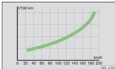
Abb. 109 Kraftstoffverbrauch in l/100 km und Geschwindigkeit in km/h
