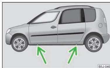
Abb. 131 Radwechsel: Aufnahmepunkte für den Wagenheber
