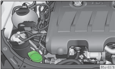
Abb. 119 Motorraum: Scheibenwaschwasserbehälter
