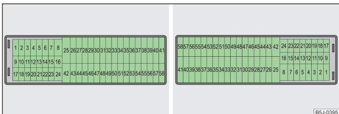
Abb. 140 Schematische Darstellung des Sicherungskastens für Links- / Rechtslenker
