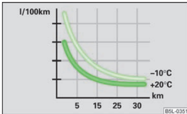
Abb. 110 Kraftstoffverbrauch in l/100 km bei verschiedenen Temperaturen
