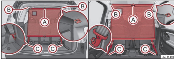
Abb. 61 Verwendung des statischen Trennnetzes hinter den Rücksitzen / hinter den vorderen Sitzen
