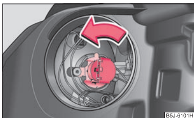
Abb. 165 Ausbau der Glühlampe für Fernlicht
