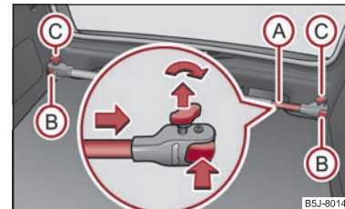
Abb. 66 Querträger einbauen
