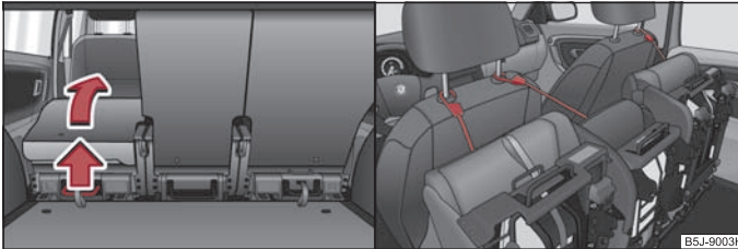
Abb. 52 Sitz komplett vorklappen / Vorgeklappte Sitze sichern
