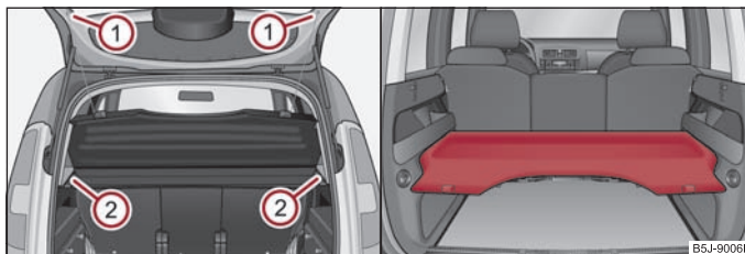
Abb. 60 Ausbau der Gepäckraumabdeckung / Gepäckraumabdeckung in der unteren Position
