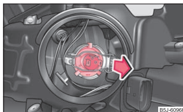
Abb. 163 Ausbau der Glühlampe für Abblend- und Fernlicht
