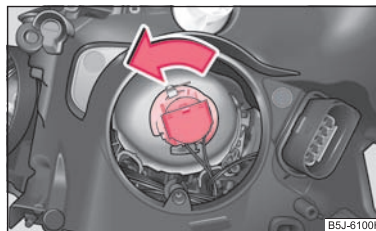
Abb. 164 Ausbau der Glühlampe für Abblendlicht
