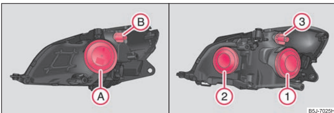
Abb. 162 Einbaulage der Lampen: Halogen-Scheinwerfer / Halogen-Projektorscheinwerfer
