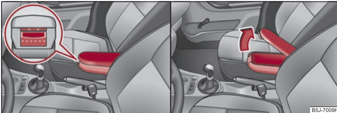
Abb. 83 Armlehne: Ablagefach / Ablagefach öffnen
