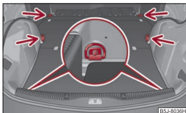
Abb. 173 Laderaum: Verzurrösen
