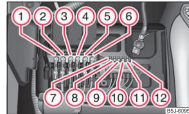
Abb. 161 Schematische Darstellung der Sicherungsbelegung an der Batterie
