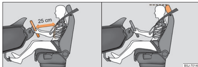
Abb. 104 Der richtige Abstand des Fahrers vom Lenkrad / die richtige Kopfstützeinstellung des Fahrers
