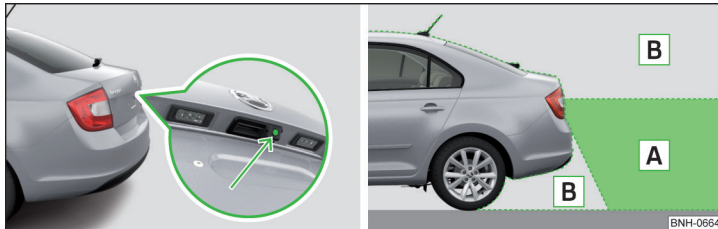
Abb. 115 Verbauplatz der Kamera / Abgetasteter Bereich hinter dem Fahrzeug
