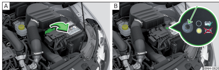
Abb. 151 Fahrzeugbatterie: Abdeckung aufklappen / Säurestandsanzeige
