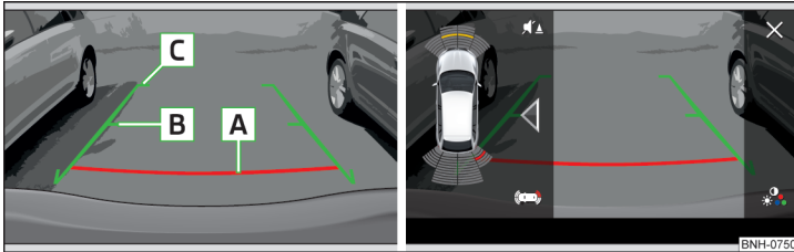
Abb. 205 Infotainmentbildschirm: Orientierungslinien / Funktionsflächen
