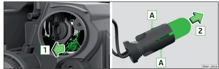
Abb. 272 Glühlampe für Standlicht wechseln
