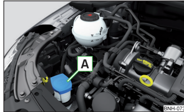
Abb. 233 Scheibenwaschwasserbehälter
