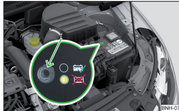
Abb. 237 Fahrzeugbatterie: Säurestands- anzeige
