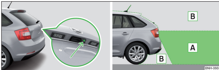
Abb. 204 Verbauort der Kamera / Abgetasteter Bereich hinter dem Fahrzeug
