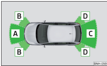
Abb. 200 Abgetastete Bereiche und Reichweite der Sensoren
