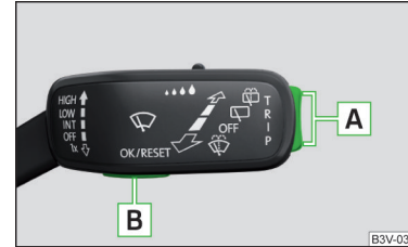
Abb. 37 Tasten am Bedienungshebel
