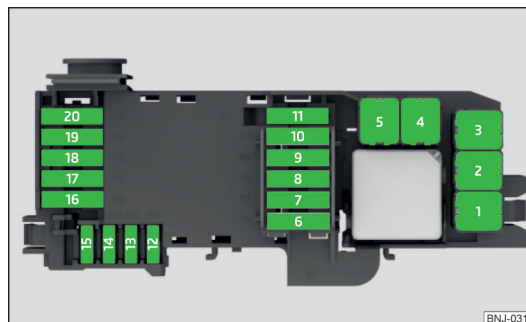
Abb. 269 Sicherungen
