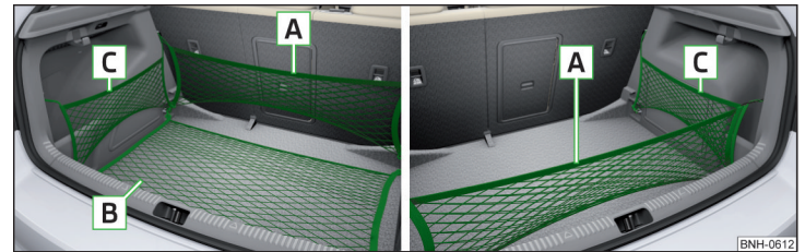
Abb. 102 Befestigungsbeispiele für Netze
