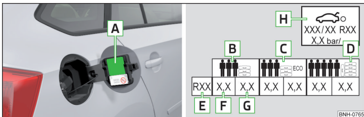
Abb. 238 Aufkleber mit einer Tabelle der Reifenfülldruckwerte / Reifen aufpumpen
