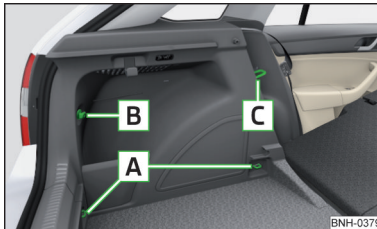
Abb. 101 Befestigungselemente
