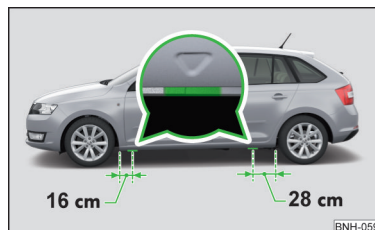
Abb. 168 Aufnahmesteg für den Wagenheber
