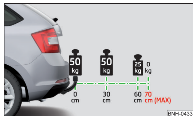
Abb. 145 Darstellung der Maximallänge des montierten Zubehörs und des zulässigen Gesamtgewichts des Zubehörs in Abhängigkeit der Ladungsschwerpunktlage
