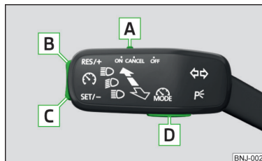
Abb. 125 Bedienelemente der Geschwindigkeitsregelanlage
