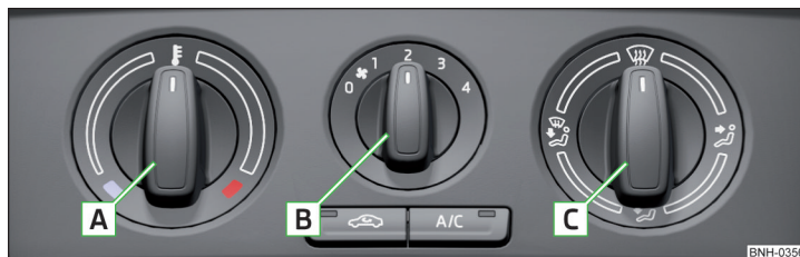
Abb. 101 Bedienelemente der Heizung/Klimaanlage
