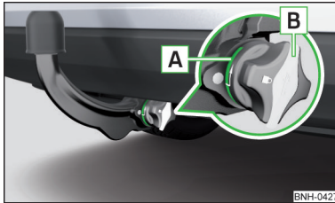
Abb. 141 Ordnungsgemäß befestigte Kugelstange
