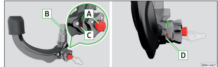
Abb. 138 Bereitschaftsstellung
