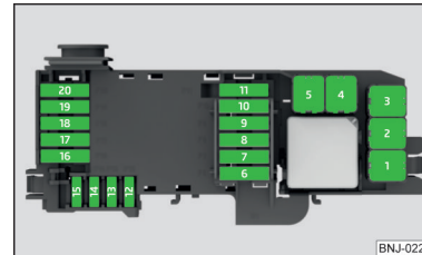
Abb. 189 Sicherungen
