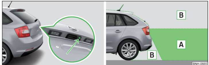
Abb. 121 Verbauport der Kamera / Abgetasteter Bereich hinter dem Fahrzeug
