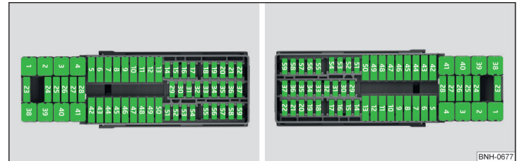
Abb. 186 Sicherungen: Linkslenkung / Rechtslenkung
