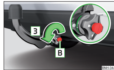
Abb. 143 Schloss entriegeln
