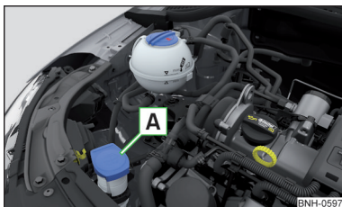
Abb. 153 Scheibenwaschwasserbehälter
