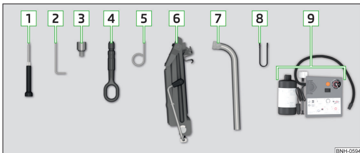
Abb. 163 Bordwerkzeug
