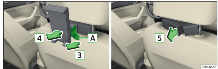
Abb. 83 Abnehmen: Halter / Adapter
