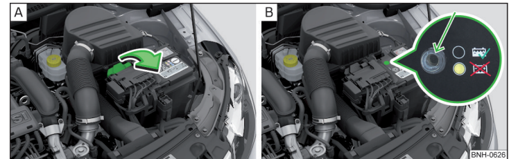
Abb. 157 Fahrzeugbatterie: Abdeckung aufklappen / Säurestandsanzeige
