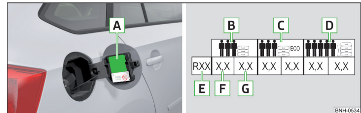
Abb. 158 Aufkleber mit einer Tabelle der Reifenfülldruckwerte / Reifen aufpumpen
