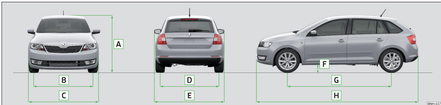
Abb. 200 Fahrzeugabmessungen
