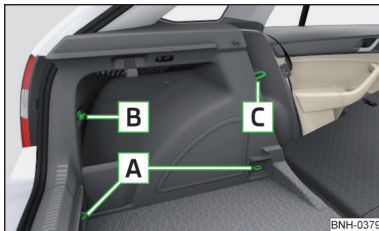
Abb. 86 Befestigungselemente
