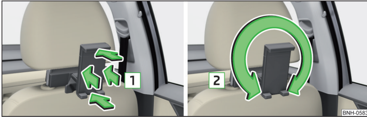
Abb. 84 Halter kippen und drehen
