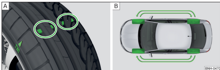
Abb. 134 Prinzipdarstellung: Reifenprofil mit Verschleißanzeigern / Rädertauschen
