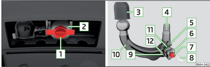
Abb. 111 Träger der Anhängervorrichtung / Kugelstange
