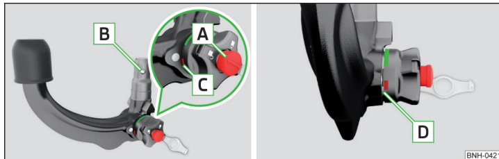
Abb. 114 Bereitschaftsstellung
