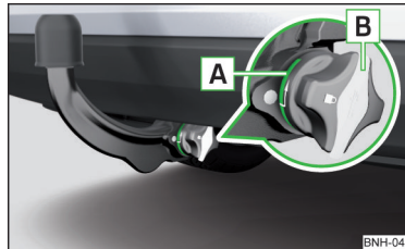
Abb. 117 Ordnungsgemäß befestigte Kugelstange
