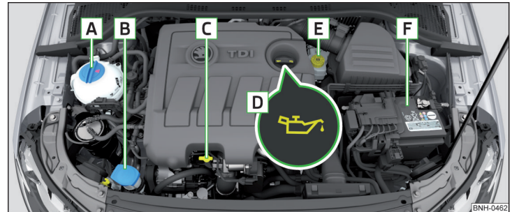
Abb. 126 Prinzipdarstellung: Motorraum
