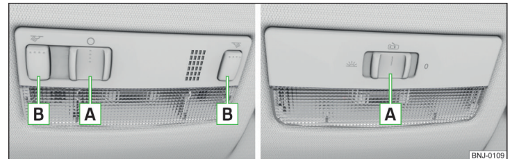
Abb. 44 Bedienung der Leuchte vorn: Variante 1 / Variante 2
