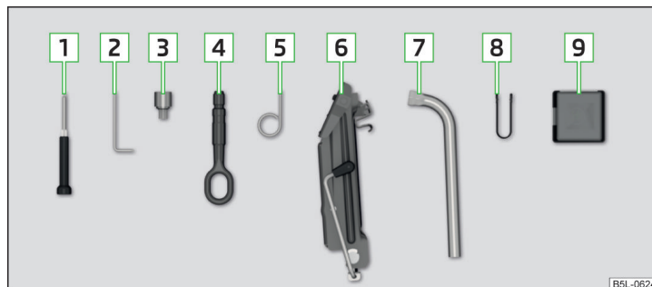
Abb. 138 Bordwerkzeug
