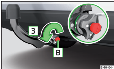
Abb. 119 Schloss entriegeln
