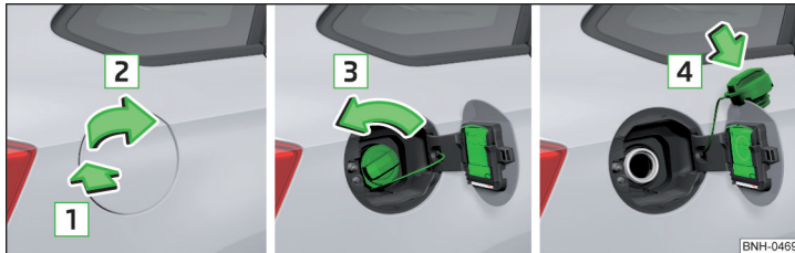
Abb. 124 Tankklappe aufklappen / Tankverschluss herausdrehen / Tankverschluss auf die Tankklappe stecken
