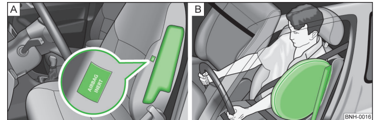
Abb. 10 Einbauort des Seitenairbags im Fahrersitz / Gasgefüllter Seitenairbag
