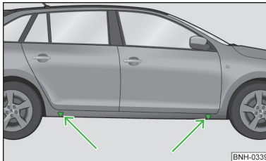
Abb. 140 Aufnahmepunkte für den Wagenheber
