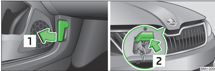
Abb. 121 Entriegelungshebel für Motorraumklappe / Entriegelungshebel
