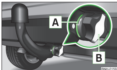
Abb. 115 Ordnungsgemäß befestigte Kugelstange
