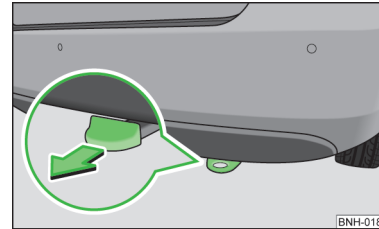
Abb. 147 Abschleppöse hinten
