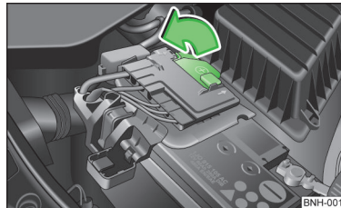
Abb. 128 Motorraum: Batterieabdeckung
