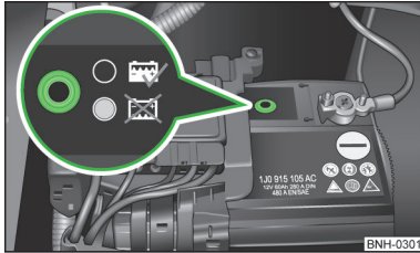
Abb. 129 Fahrzeugbatterie: Säurestands- anzeige
