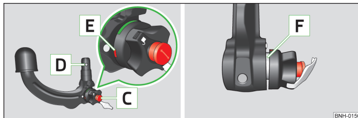
Abb. 112 Bereitschaftsstellung
