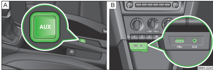
Abb. 97 AUX-Eingang / MDI-Eingang
