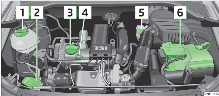
Abb. 123 Prinzipdarstellung: Motorraum
