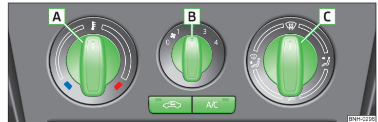
Abb. 92 Bedienelemente der Klimaanlage
