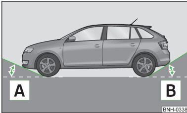
Abb. 171 Prinzipdarstellung: Überhangwinkel
