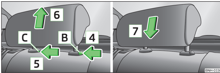
Abb. 53 Kopfstütze hinten aus-/einbauen
