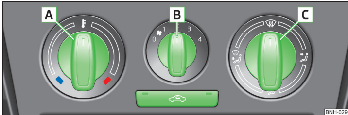
Abb. 91 Heizungsbedienelemente
