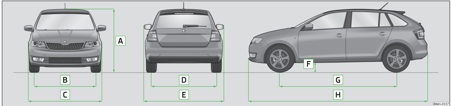
Abb. 170 Prinzipdarstellung: Fahrzeugabmessungen
