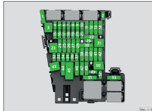
Abb. 354 Sicherungen
