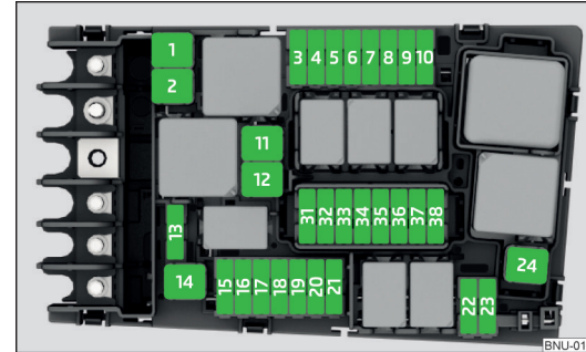
Abb. 356 Sicherungen
