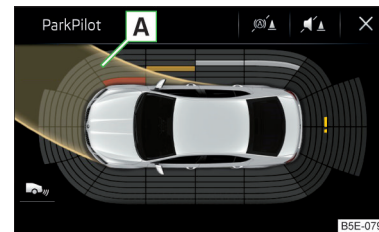
Abb. 256 Bildschirmanzeige
