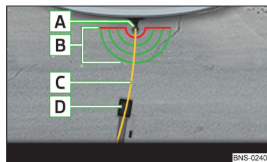
Abb. 269 Bildschirmanzeige
