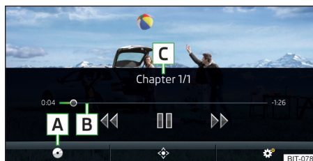
Abb. 188 Video-DVD: Hauptmenü
