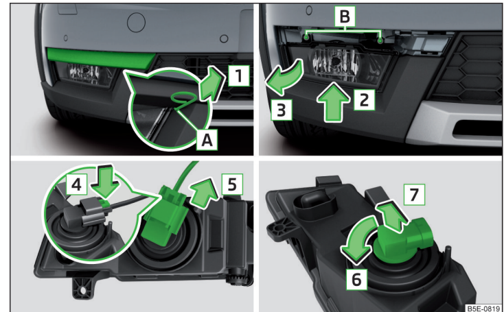
Abb. 360 Nebelscheinwerfer herausnehmen / Glühlampe wechseln - Variante 2
