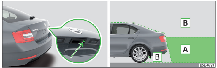
Abb. 260 Verbauort der Kamera / Abgetasteter Bereich hinter dem Fahrzeug
