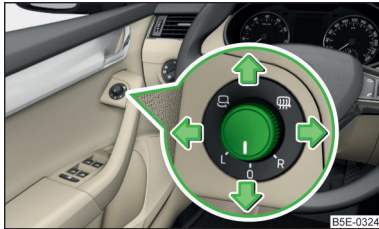
Abb. 78 Außenspiegelbedienung
