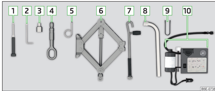
Abb. 327 Bordwerkzeug
