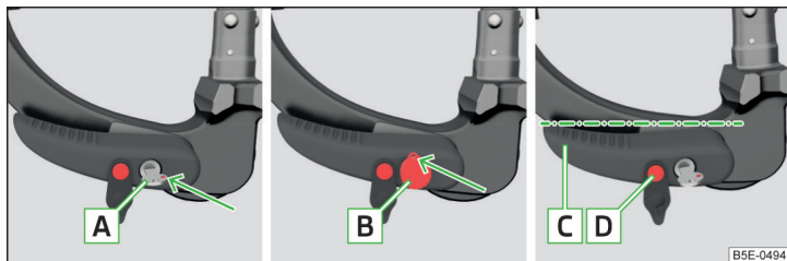
Abb. 300 Bereitschaftsstellung: Schlüsselvariante 1 / Schlüsselvariante 2 / Stellung des Hebels und des Auslösebolzens bei beiden Schlüsselvarianten
