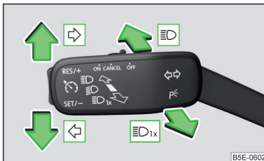
Abb. 63 Bedienungshebel: Blink- und Fernlichtbedienung
