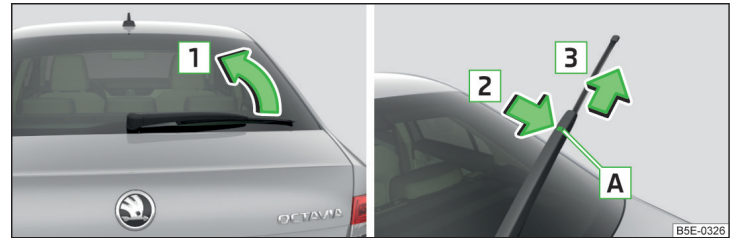
Abb. 349 Scheibenwischerblatt der Heckscheibe auswechseln
