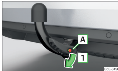
Abb. 305 Kappe vom Schloss abnehmen
