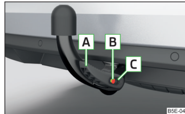
Abb. 304 Ordnungsgemäß befestigte Ku- gelstange
