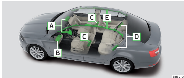
Abb. 19 Verbaute der Airbags
