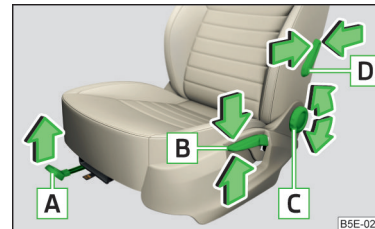
Abb. 79 Bedienelemente am Sitz
