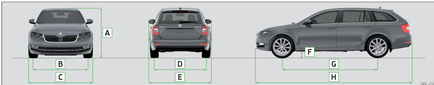
Abb. 367 Fahrzeugabmessungen
