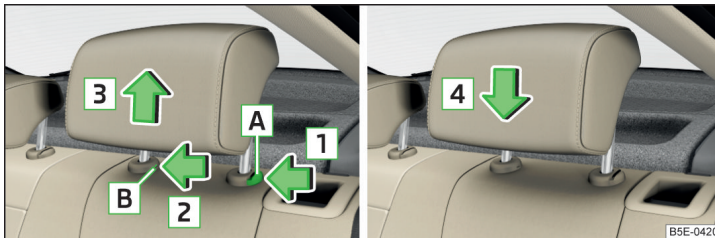
Abb. 89 Kopfstütze hinten herausnehmen/einsetzen
