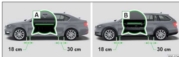
Abb. 332 Aufnahmesteg für den Wagenheber: Variante 1 / Variante 2
