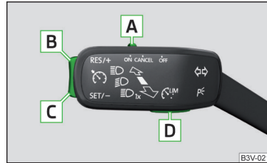
Abb. 279 Bedienelemente des Geschwindigkeitsbegrenzers (Variante mit GRA)
