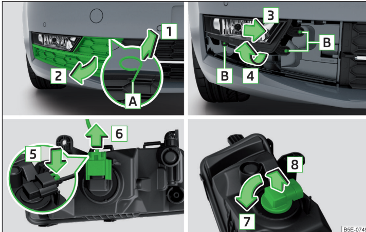
Abb. 359 Nebelscheinwerfer herausnehmen / Glühlampe wechseln - Variante 1
