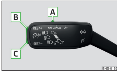
Abb. 297 Bedienelemente des Geschwindigkeitsbegrenzers (Variante ohne GRA)
