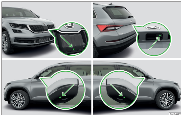
Abb. 282 Verbauorte der Kameras für die Umgebungserfassung
