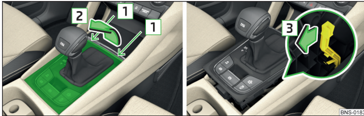
Abb. 357 Abdeckung lösen / Wählhebel entriegeln
