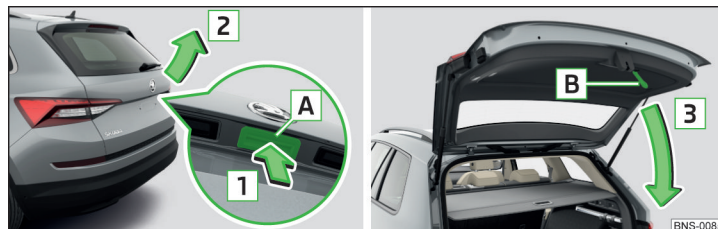
Abb. 58 Gepäckraumklappe öffnen/schließen
