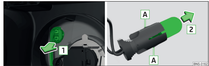
Abb. 369 Glühlampe für Standlicht wechseln
