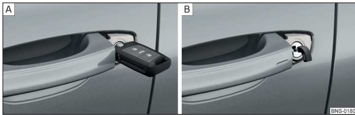
Abb. 354 Griff an der Fahrertür: Schlüssel mit herausklappbarem Schlüsselbart / KESSY-Notschlüssel
