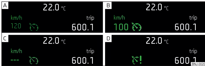
Abb. 294 Display des Kombi-Instruments: Beispiele für Zustandsanzeigen der GRA
