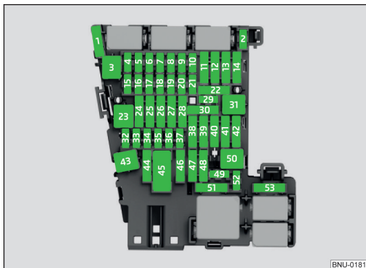
Abb. 364 Sicherungen
