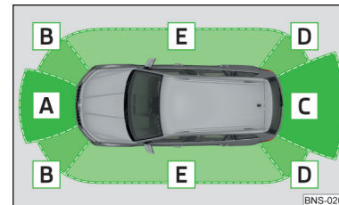
Abb. 267 Abgetastete Bereiche und Reichweite der Sensoren
