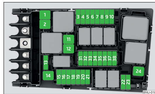
Abb. 366 Sicherungen
