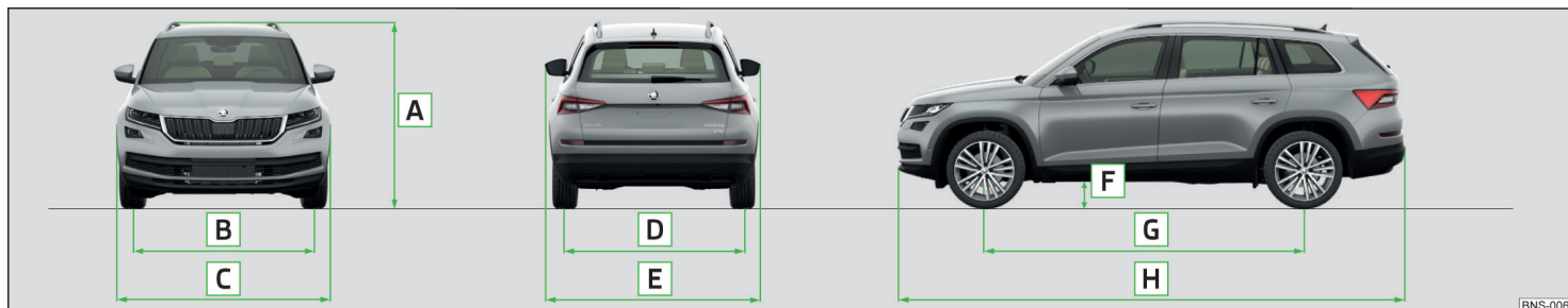
Abb. 378 Fahrzeugabmessungen
