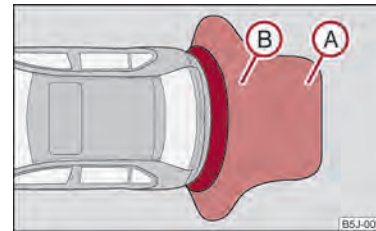
Abb. 85 Einparkhilfe: Reichweite der Sensoren
