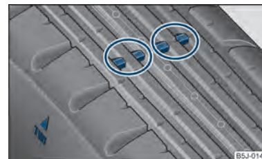
Abb. 136 Reifenprofil mit Verschleißanzeiger
