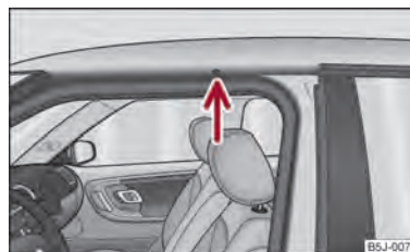
Abb. 60 Befestigungspunkte für Grunddachträger
