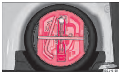
Abb. 138 Gepäckraum: Ablage für das Bordwerkzeug
