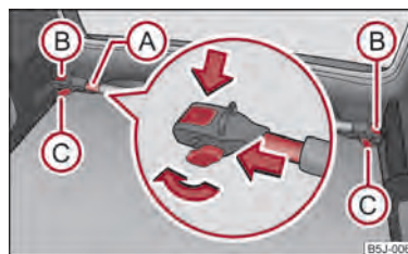
Abb. 56 Querträger einbauen
