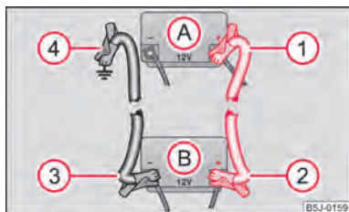
Abb. 147 Starthilfe mit der Batterie eines anderen Fahrzeugs: A - entladene Fahrzeugbatterie, B - stromgebende Batterie
