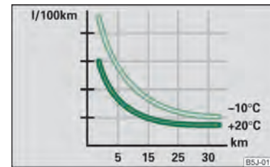
Abb. 123 Kraftstoffverbrauch in l/100 km bei verschiedenen Temperaturen
