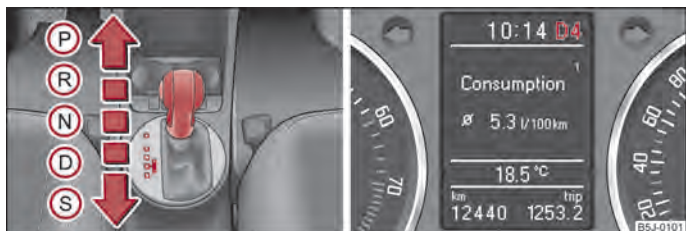
Abb. 88 Wählhebel / Informationsdisplay: Wählhebelstellungen
