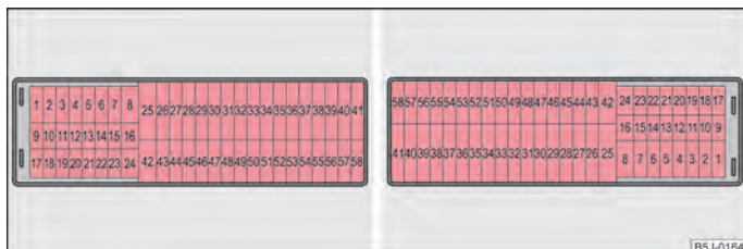
Abb. 152 Schematische Darstellung der Sicherungsbox für Links- / Rechtslenkfahrzeuge
