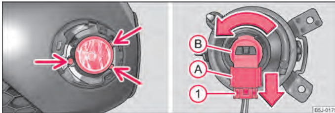
Abb. 163 Vorderer Stoßfänger: Nebelscheinwerfer / Lampenwechsel
