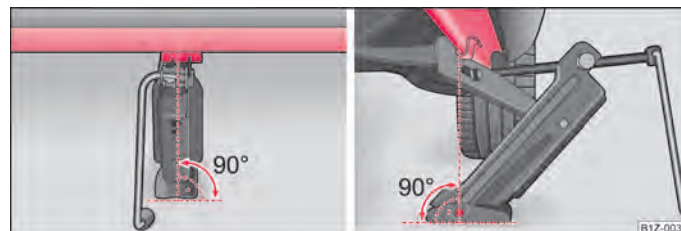
Abb. 144 Wagenheber ansetzen
