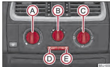
Abb. 79 Klimaanlage: Bedienelemente
