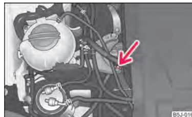
Abb. 148 Starthilfe bei Fahrzeugen mit START-STOPP-System ▶
