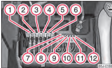
Abb. 156 Schematische Darstellung der Sicherungsbelegung an der Batterie
