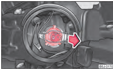
Abb. 158 Ausbau der Glühlampe für Abblend- und Fernlicht
