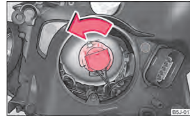
Abb. 159 Ausbau der Glühlampe für Abblend- und Fernlicht / Abblendlicht
