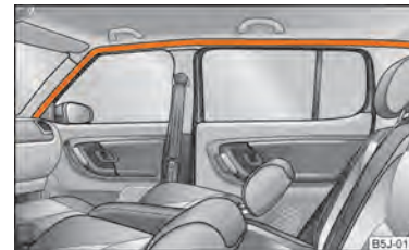
Abb. 107 Einbauorte des Kopf-Airbags
