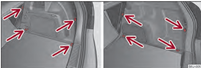
Abb. 44 Gepäckraum: Verzurrösen und Befestigungselemente (Fabia) / (Combi)
