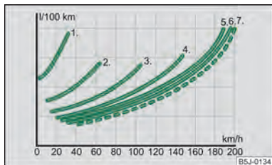
Abb. 121 Kraftstoffverbrauch in l/100 km und Geschwindigkeit in km/h
