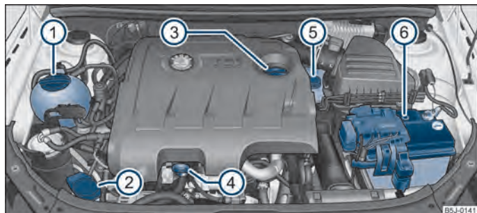
Abb. 128 Dieselmotor 1,6 l/77 kW
