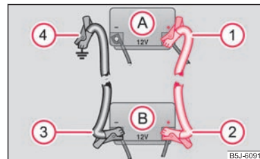
Abb. 159 Starthilfe mit der Batterie eines anderen Fahrzeugs: A - entladene Fahrzeugbatterie, B - stromgebende Batterie
