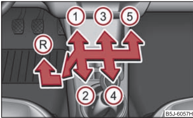
Abb. 96 Schaltschema bei Fahrzeugen mit 5-Gang Schaltgetriebe
