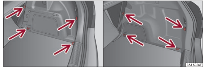
Abb. 57 Kofferraum: Verzurrösen und Befestigungselemente (Fabia) / (Combi)
