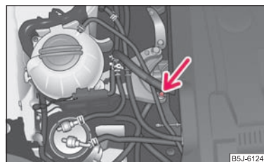
Abb. 160 Starthilfe bei Fahrzeugen mit START-STOPP-System
