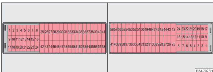
Abb. 164 Schematische Darstellung der Sicherungsbox für Links- / Rechtslenkerfahrzeuge
