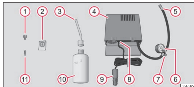
Abb. 158 Bestandteile des Reifenreparatursets
