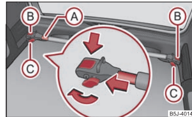
Abb. 69 Querträger einbauen
