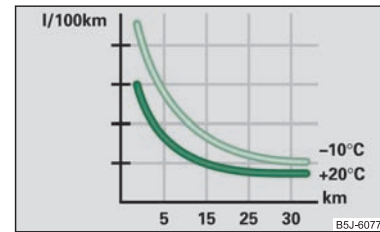
Abb.136 Kraftstoffverbrauch in l/100 km bei verschiedenen Temperaturen
