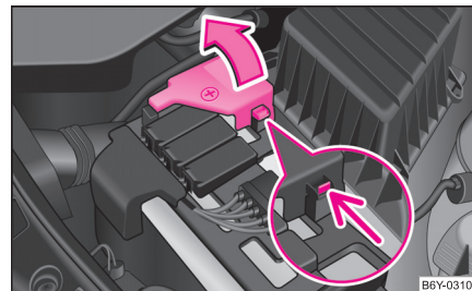
Abb. 174 Batterie: Abdeckung aufklappen
