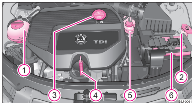
Abb. 170 Dieselmotor 1,9 l/77 kW
