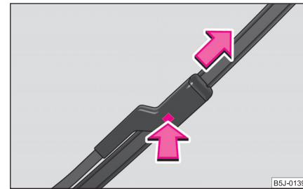
Abb. 46 Wischerblatt für Frontscheibe
