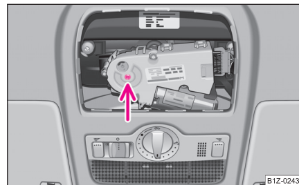
Abb. 32 Ausschnitt des Dachhimmels: Notbetätigung
