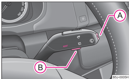
Abb. 6 Multifunktionsanzeige: Bedienelemente
