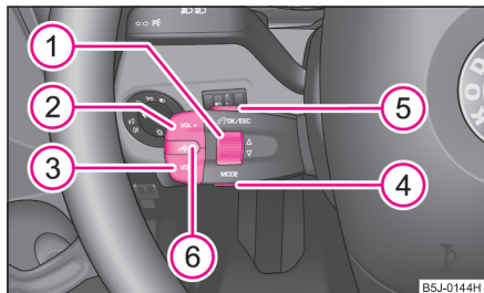
Abb. 123 Multifunktionsmodul: Tasten für die Radio- und Telefonbedienung
