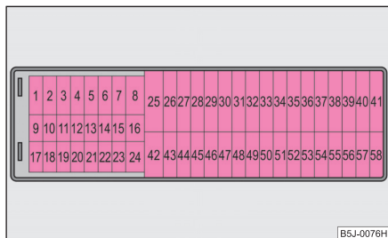
Abb. 193 Schematische Darstellung der Sicherungsbox für Linkslenkfahrzeuge.
