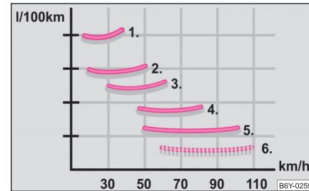
Abb. 162 Kraftstoffverbrauch in l/100 km und Geschwindigkeit in km/h
