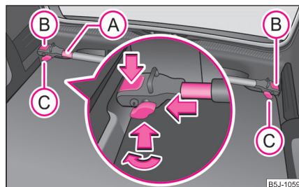
Abb. 78 Querträger einbauen
