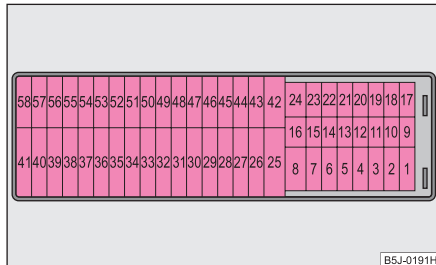
Abb. 194 Schematische Darstellung der Sicherungsbox für Rechtslenkfahrzeuge.
