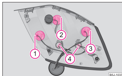
Abb. 207 Heckleuchteinheit: Einbaulage der Glühlampen
