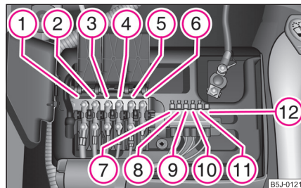
Abb. 197 Schematische Darstellung der Sicherungs- belegung an der Batterie
