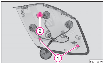
Abb. 206 Heckleuchteinheit einbauen
