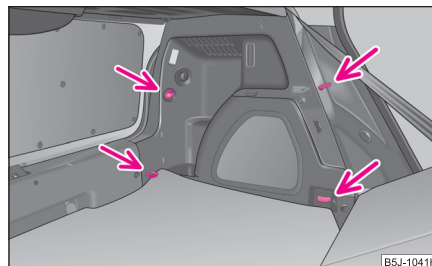
Abb. 57 Gepäckraum: Verzurrösen und Verzurrhaken (Fabia)
