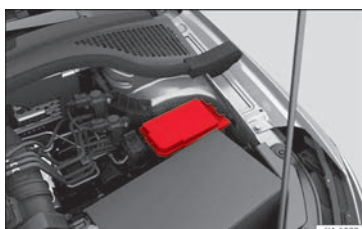
Abb. 56 Im Motorraum: Abdeckung des Sicherungskastens.
