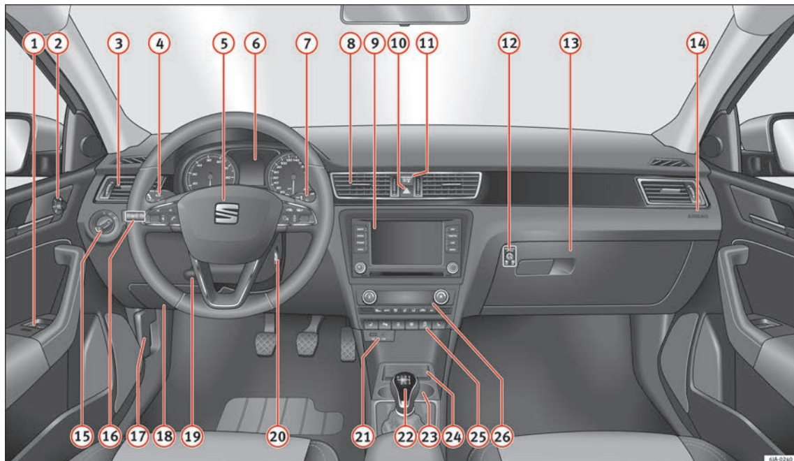
Abb. 110 Fahrzeuginnenraum
