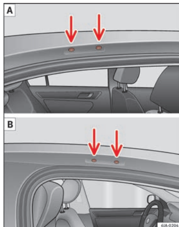
Abb. 168 Befestigungspunkte für Grundträger
