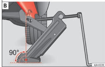
Abb. 65 Wagenheber anbringen
