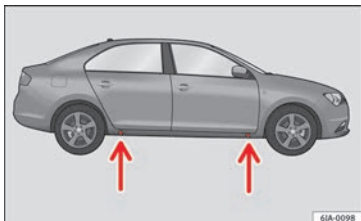
Abb. 64 Radwechsel: Ansetzstellen für den Wagenheber
