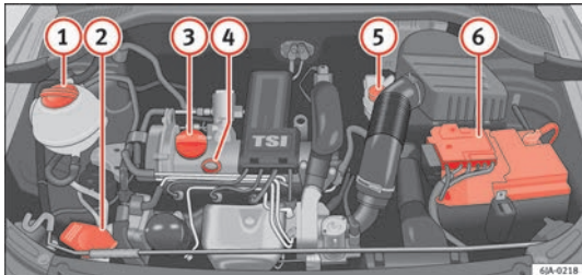
Abb. 205 Abbildung für die Einbaustellen der Elemente
