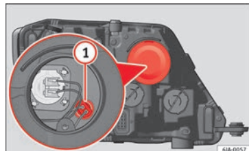
Abb. 90 Glühlampe für Standlicht auswechseln
