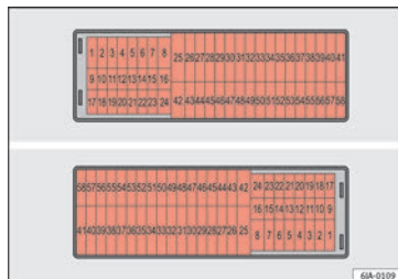
Abb. 86 Schematische Darstellung des Sicherungskastens links/rechts vom Lenkrad.
