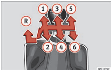
Abb. 177 Schaltschema des 5- bzw. 6-Gang-Schaltgetriebes
