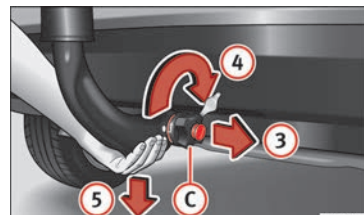
Abb. 201 Kugelkopfstange entriegeln
