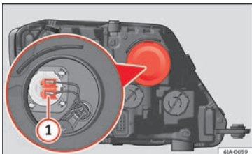
Abb. 91 Glühlampe für Fernlicht auswechseln
