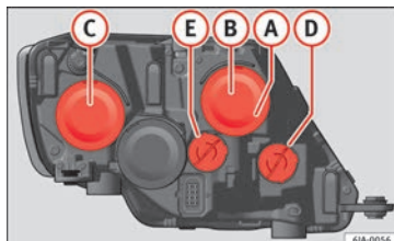
Abb. 89 Glühlampen des Hauptscheinwerfers
