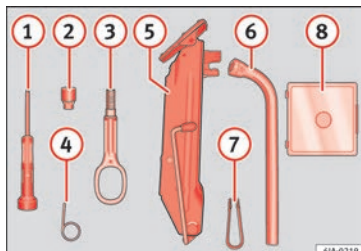
Abb. 59 Bordwerkzeug
