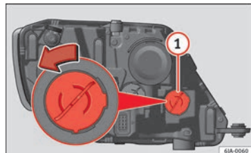
Abb. 94 Glühlampe für Blinklicht auswechseln
