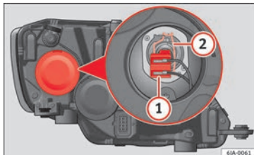
Abb. 93 Glühlampe für Ablendlicht auswechseln
