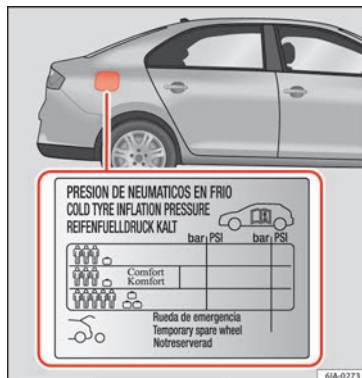
Abb. 213 Einbauort des Aufklebers für den Reifenfülldruck.
