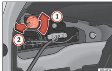
Abb. 116 Lampenhalter ausbauen.
