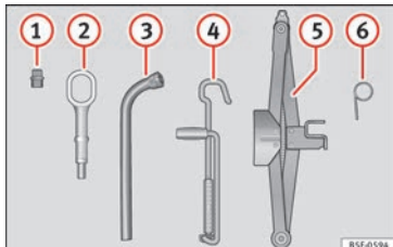
Abb. 68 Im Gepäckraum unter dem Gepäckraumboden: Bordwerkzeug.
