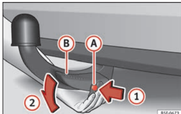
Abb. 235 Abnehmbaren Kugelkopf lösen
