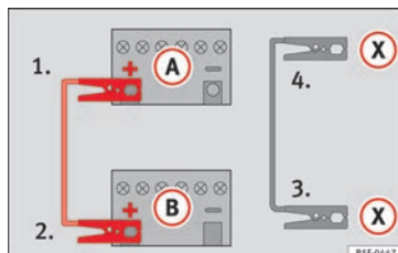
Abb. 78 Anschlussschema für Fahrzeuge mit Start-Stopp-System.
