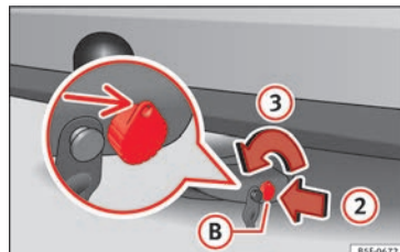
Abb. 234 Schloss entriegeln
