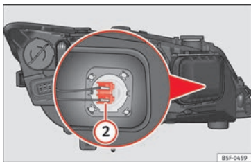
Abb. 108 Fernlichtleuchte.
