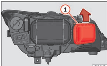
Abb. 107 Fernlichtleuchte.
