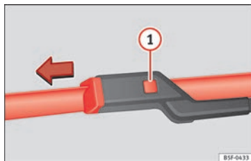
Abb. 80 Scheibenwischerblätter vorne austauschen.
