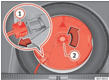
Abb. 249 Im Gepäckraum: Subwoofer ausbauen.
