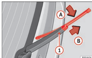
Abb. 81 Scheibenwischerblatt der Heckscheibe austauschen.
