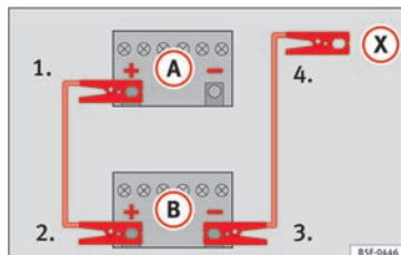
Abb. 77 Anschlussschema für Fahrzeuge ohne Start-Stopp-System.
