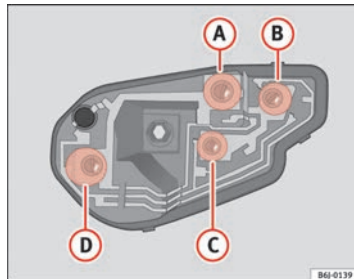
Abb. 161 Leuchte rechts
