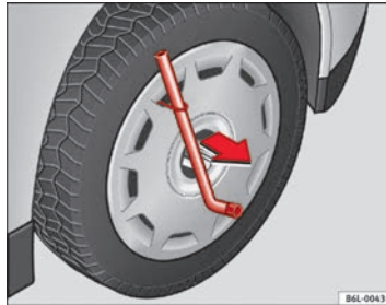
Abb. 135 Die Radvollblende vom Rad abnehmen
