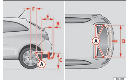
Abb. 117 Befestigungspunkte für die Anhängervorrichtung
