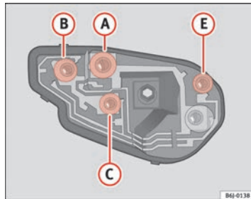
Abb. 160 Leuchte links
