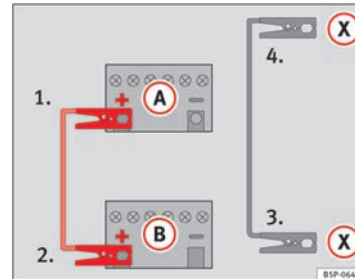
Abb. 170 Schaltschema zum Anschluss der Starthilfekabel, falls das stromgebende Fahrzeug mit einem Start-Stopp-System ausgestattet ist: entladene Batterie (A) und stromgebende Batterie (B).
