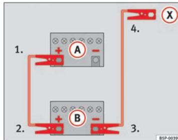
Abb. 169 Schaltschema zum Anschluss des Starthilfekabel, falls das stromgebende Fahrzeug über kein Start-Stopp-System verfügt: entladene Batterie (A) und stromgebende Batterie (B).
