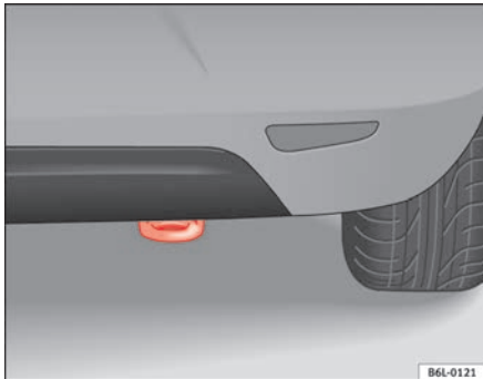
Abb. 175 Hintere Abschleppöse
