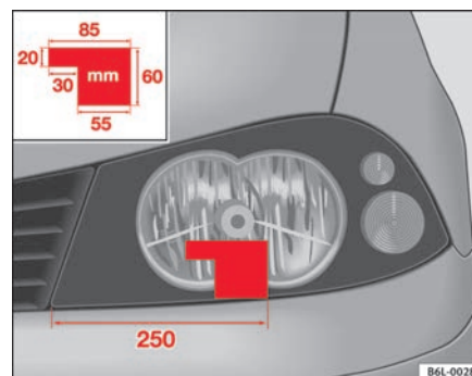
Abb. 112 Linker Scheinwerfer
