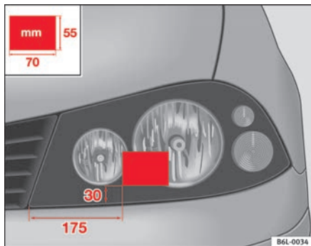
Abb. 118 Linker Scheinwerfer
