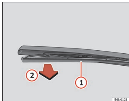
Abb. 132 Scheibenwischerblatt hinten auswechseln
