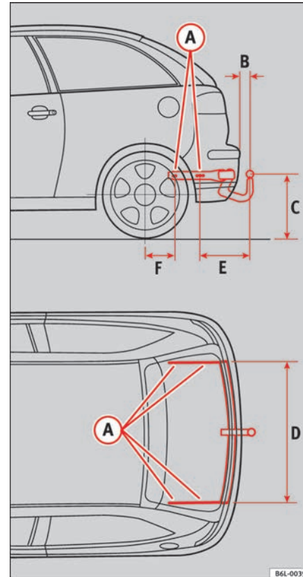
Abb. 123 Befestigungspunkte für die Anhangvorrichtung
