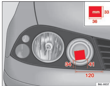
Abb. 121 Rechter Scheinwerfer
