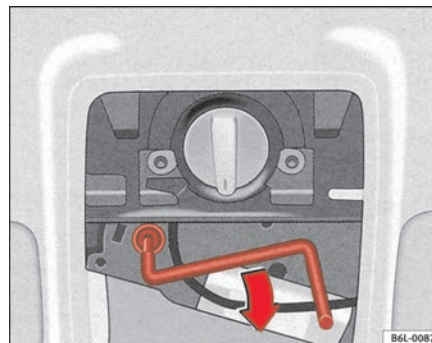
Abb. 56 Kurbel für Notverriegelung
