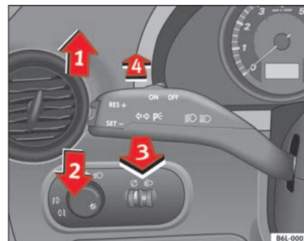
Abb. 61 Blinker und Fernlichthebel
