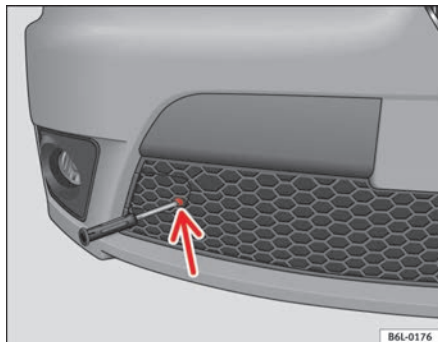
Abb. 172 Deckel der Abschleppöse unten am mittleren Gitter
