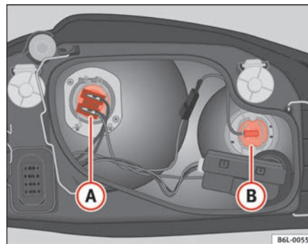
Abb. 148 Glühlampe des Hauptscheinwerfers
