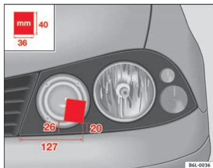
Abb. 120 Linker Scheinwerfer
