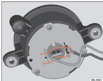
Abb. 159 Nebelscheinwerfer
