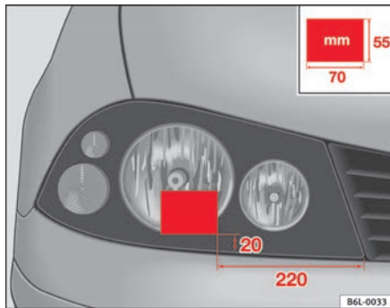
Abb. 117 Rechter Scheinwerfer
