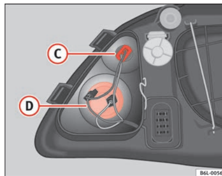
Abb. 149 Glühlampe des Hauptscheinwerfers
