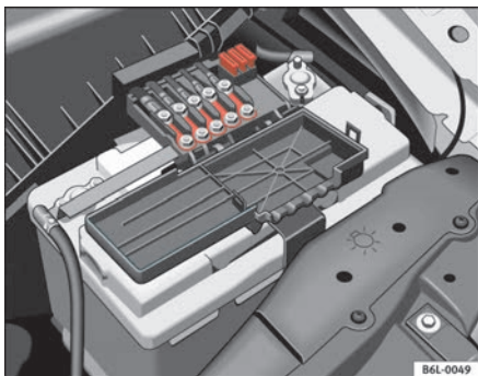
Abb. 147 Sicherungskasten auf Batterie
