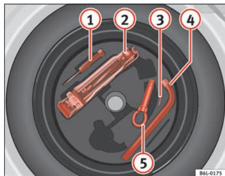
Abb. 136 Werkzeugbox
