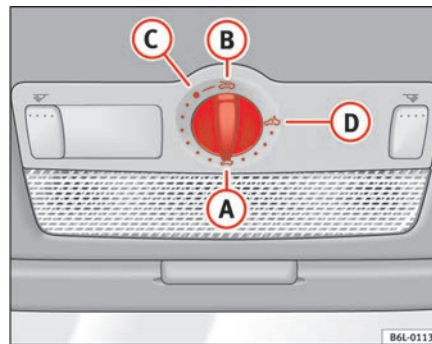
Abb. 55 Ausschnitt aus dem Dachhimmel: Drehschalter Schiebe-/Ausstelltdach
