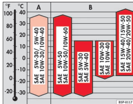
Abb. 126 Öltypen nach Temperaturbereichen
