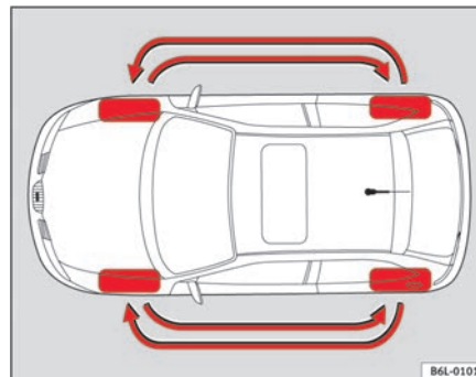
Abb. 135 Schema für das Tauschen der Räder
