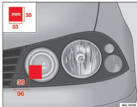
Abb. 122 Linker Scheinwerfer
