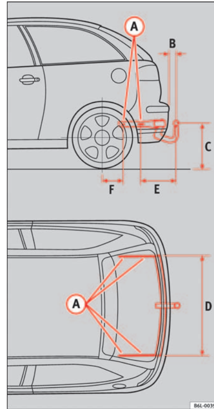
Abb. 118 Befestigungspunkte für die Anhangvorrichtung
