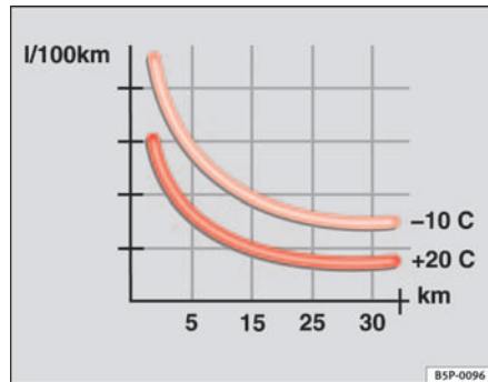
Abb. 117 Kraftstoffverbrauch in l/100km bei zwei verschiedenen Umgebungstemperaturen
