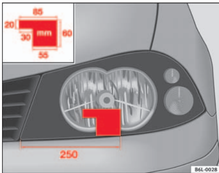
Abb. 106 Linker Scheinwerfer
